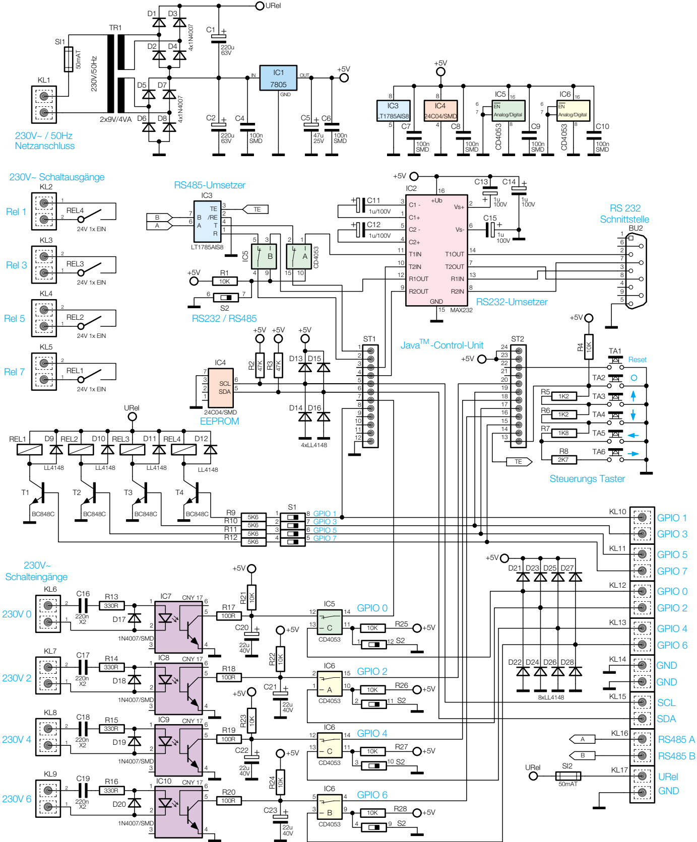
Bild 1: Schaltbild des Schaltinterfaces JCU10 SI
