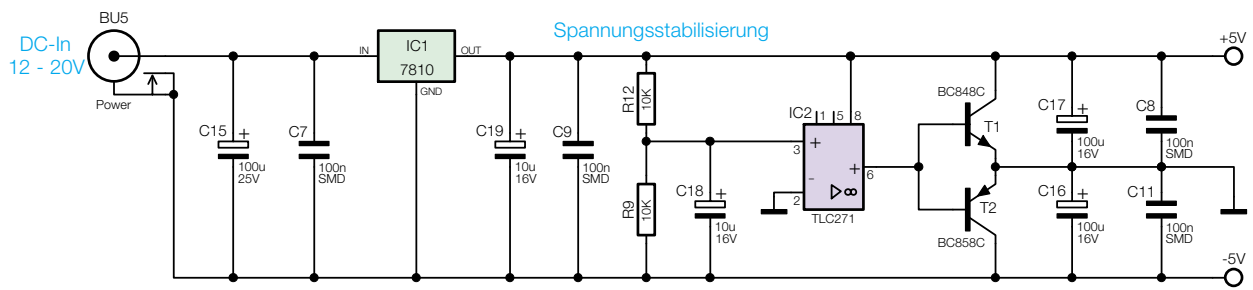
Bild 2: Schaltbild der SBV 1
