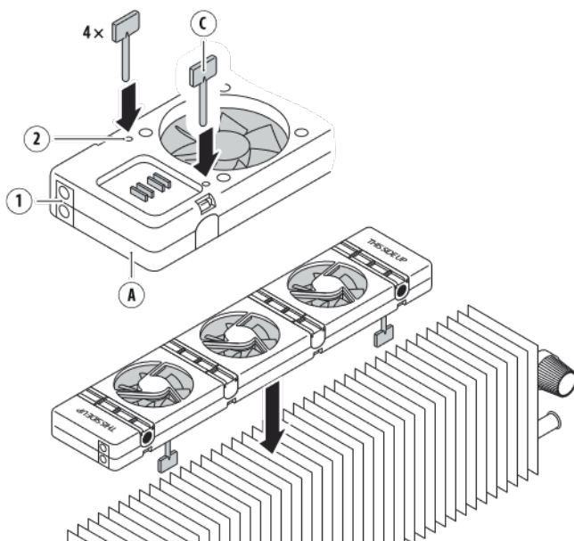
Fig. 8 - Fixation d'un pied (C).
