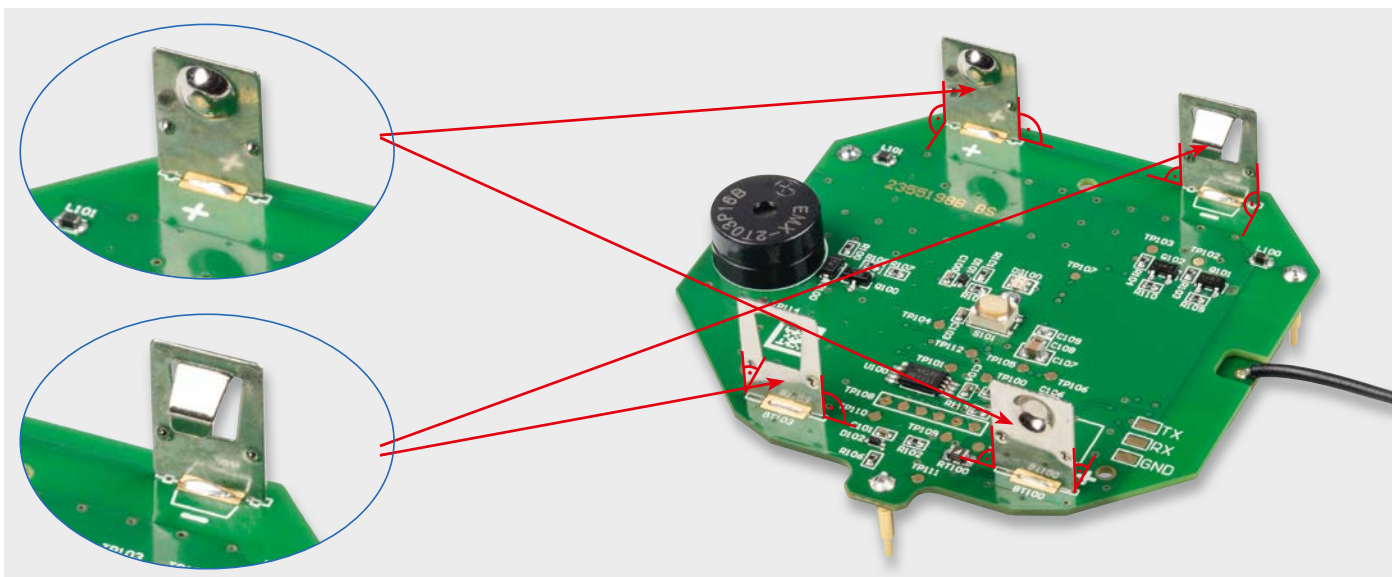
Bild 6: Die Batteriekontakte werden rechtwinklig und bündig verlötet.
