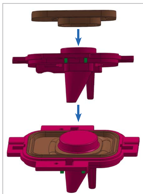
Bild 10: Zusammensetzung des Lichtleiters und der Dichtung (3D-Zeichnung)
