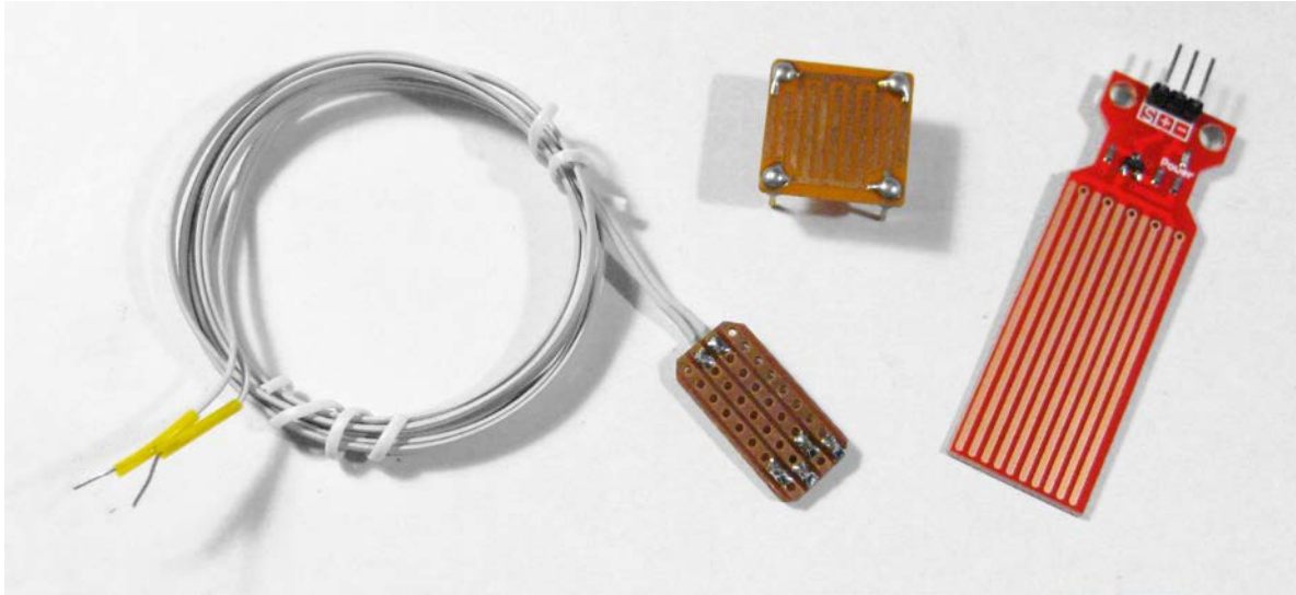
Bild 1: Selbst gebaute (links) und kommerzielle (rechts) Feuchtesensoren
