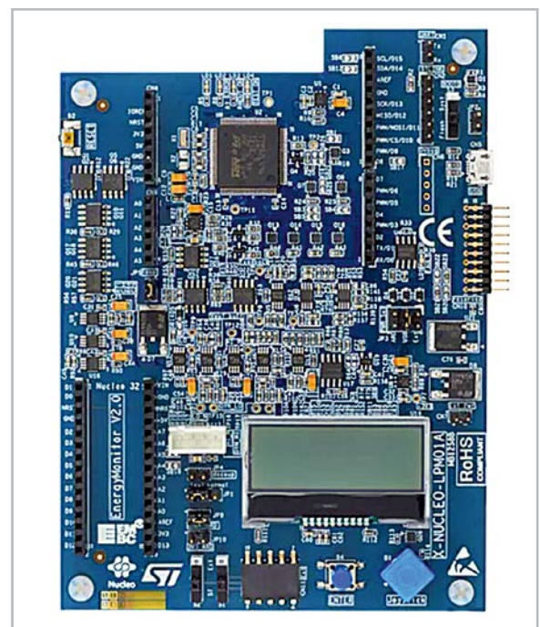
Bild 6: Erweiterungsboard für Energiemessungen ST X-NUCLEO-LPM01A
