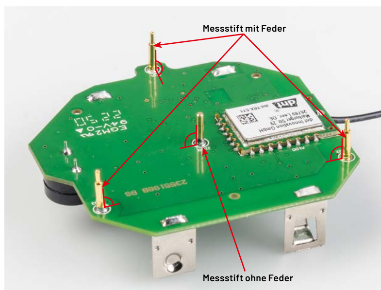
Bild 7: Die Messstifte werden rechtwinklig und bündig verlötet (in der Mitte wird der Messstift ohne Feder verwendet).
