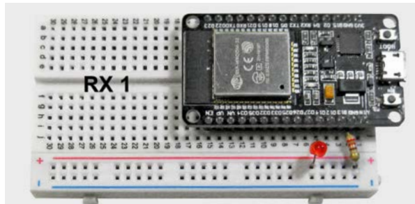
Bild 9: Die beiden identischen Empfänger können individuell geschaltet werden.
