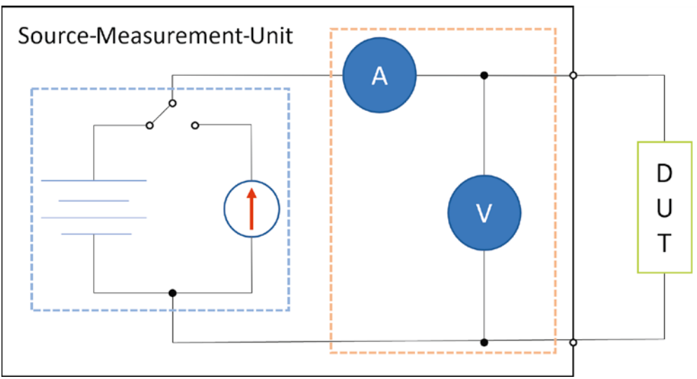
Bild 2: Schematischer Aufbau einer Source-Measure-Unit nach [9]
