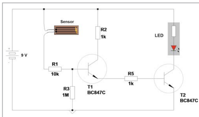
Bild 3: Schaltung zum Regenmelder
