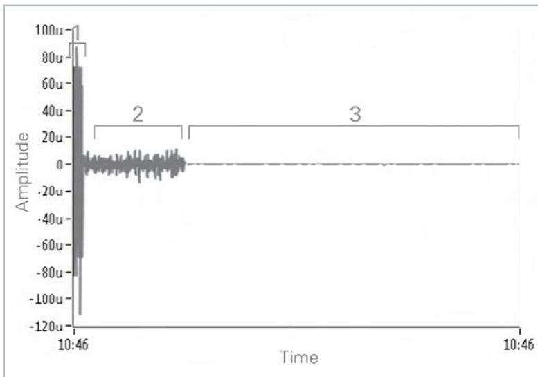
Bild 5: Auswirkung der Blendzeit auf das Messrauschen aus [10]
