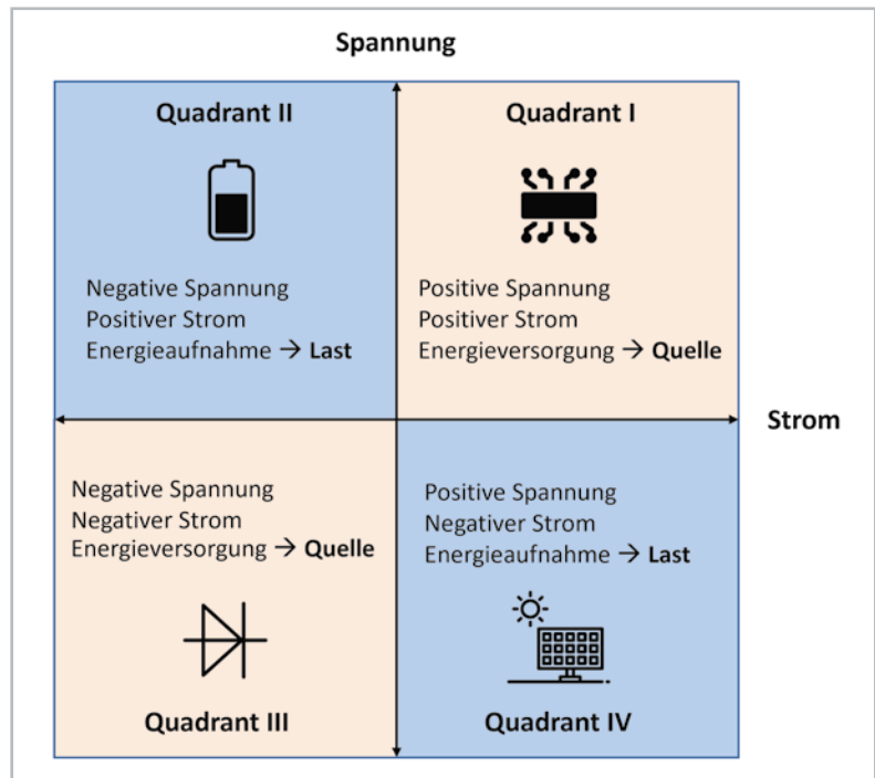
Bild 3: Operationsbereich von Sourcemetern im 4-Quadranten-Modell nach [2]
