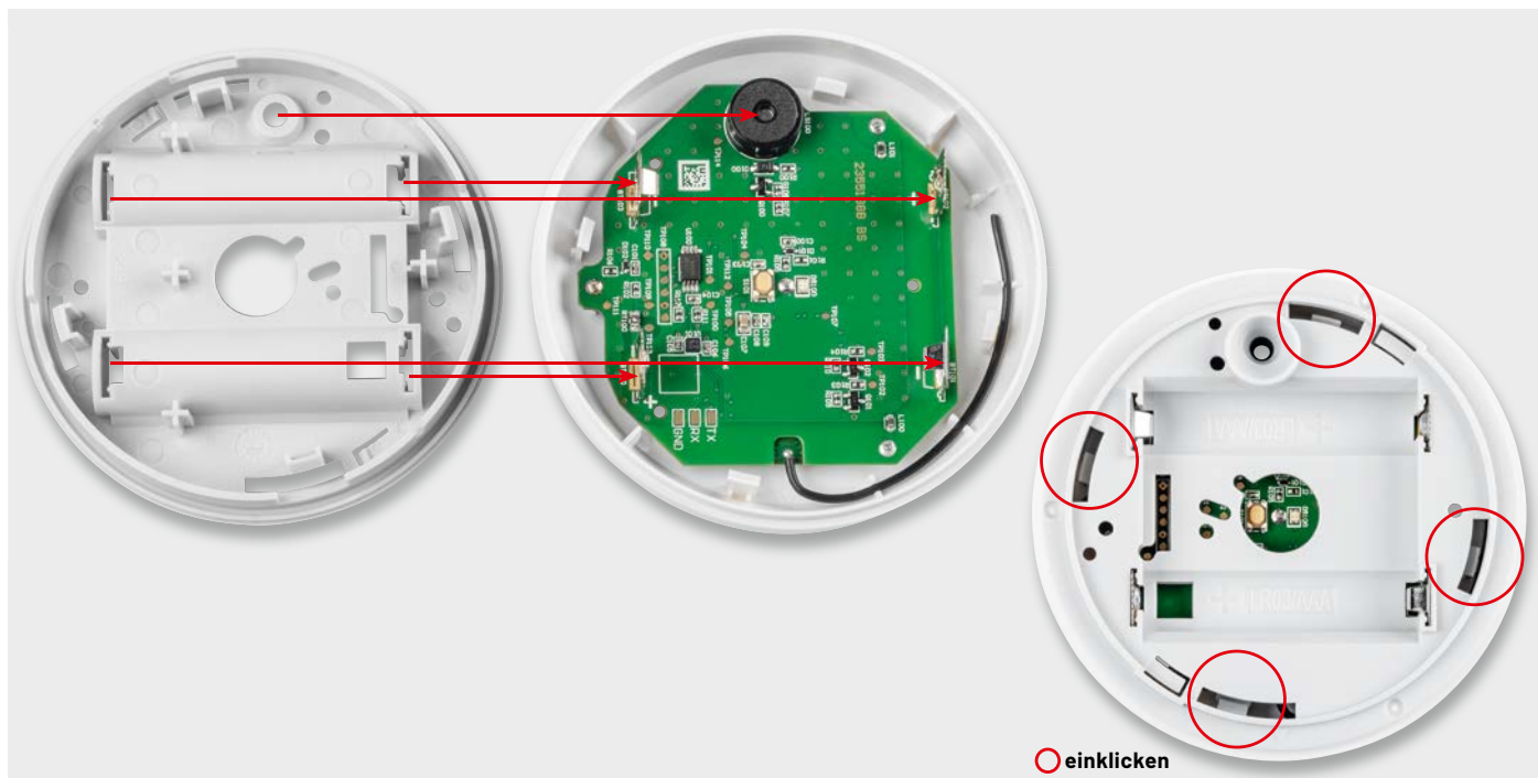
Bild 16: Einsetzen des Gehäusekerns (links, Signalgeber dient als Hinweis für die Ausrichtung) und fertig eingeklickter Gehäusekern (rechts)
