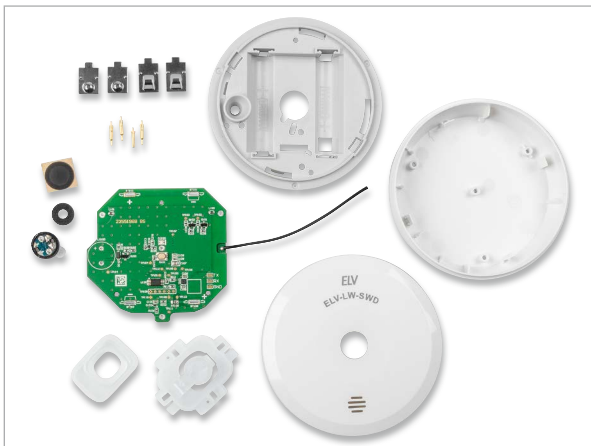
Bild 3: Lieferumfang des ELV LoRaWAN® Wassersensors
