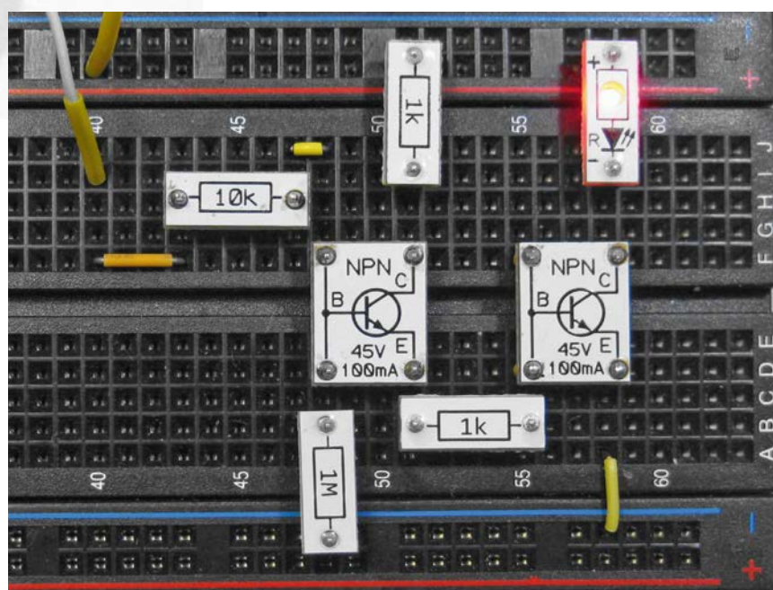
Bild 4: Aufbau zur Regenmelderschaltung
