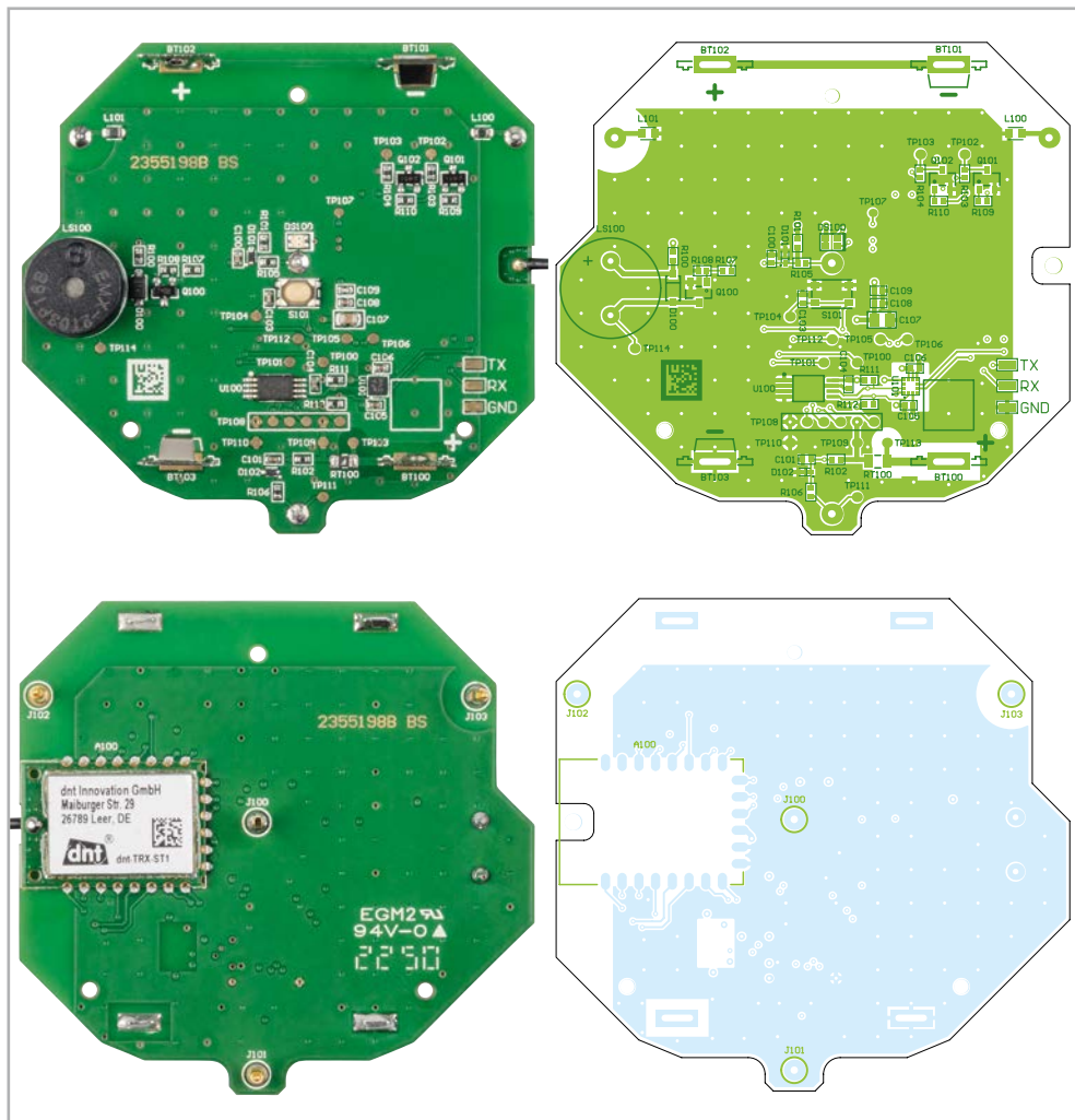
Bild 4: Platinfotos und Bestückungsdrucke des ELV-LW-SWD
