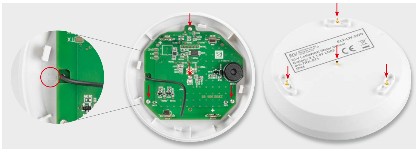
Bild 12: Pfeil als Hilfsmarkierung für die Ausrichtung der PCB (links), Leiterplatte in der Gehäuseunterschale eingesetzt (Mitte) und die Messstifte des Geräts nach dem Einsetzen der Leiterplatte (rechts)
