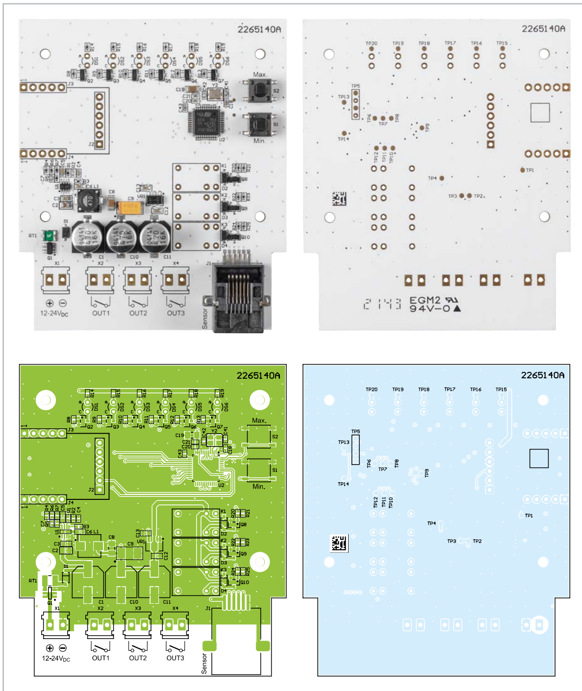
Bild 5: Platinenfotos und Bestückungsdrucke der Anzeigeinheit
