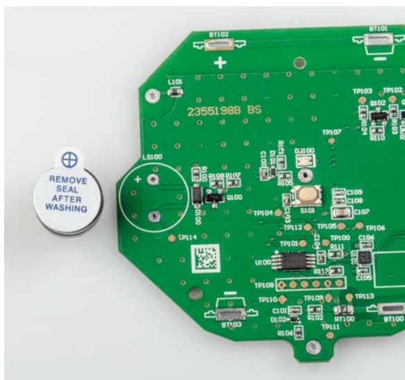
Bild 5: Gekennzeichnete Polarität auf der PCB und dem Signalgeber
