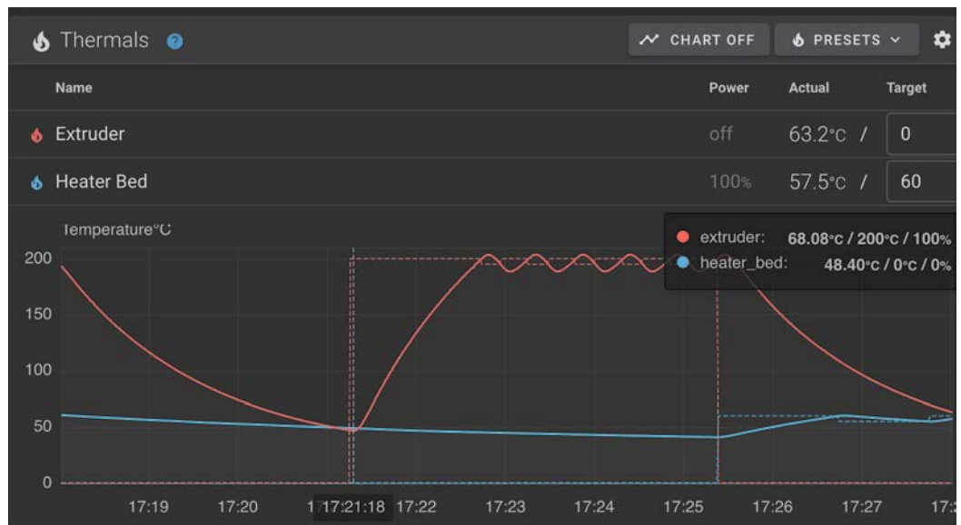
Bild 15: Die Konfigurationsdatei lässt sich über den integrierten Editor sehr einfach anpassen. Hier ist das Regelverhalten der Extruderheizung (PID) und der ermittelte Wert für „Pressure Advance“ eingetragen.
