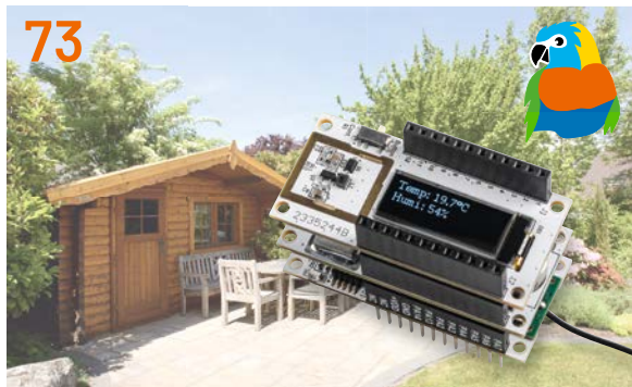
Applikationsmodul Display 1 für LoRaWAN®
