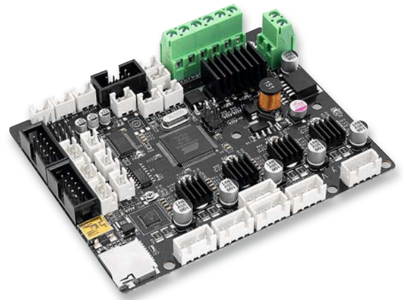
Bild 2: Moderne Motherboards, hier das aktuelle Silent Motherboard von Creality, fassen die gesamte Steuerung auf einer kompakten Platine zusammen. Diese Bauform ist heute die Norm. Bild: Creality
