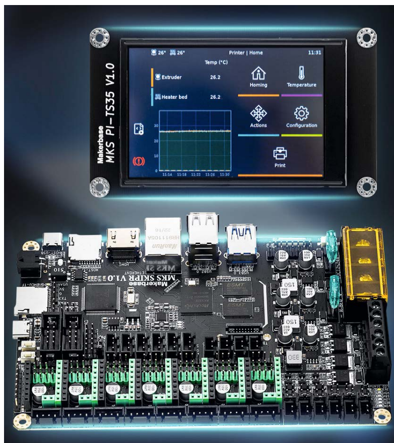
Bild 9: Das SKIPR-Board von Makerbase ist, samt Touchdisplay, eine komplette DIY-Nachrüstlösung. Bild: Makerbase
