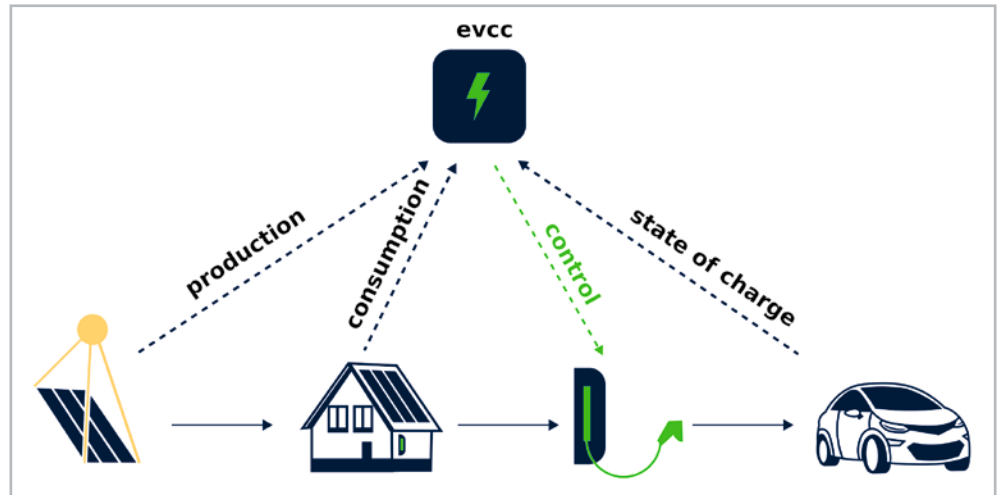
Bild 1: Informationsfluss und Funktionsweise von evcc [1]
