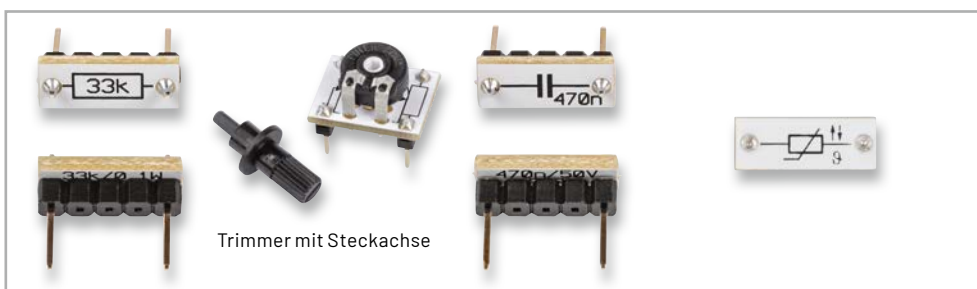
Bild 23: Widerstand, Potentiometer, Kondensator und NTC-Widerstand
