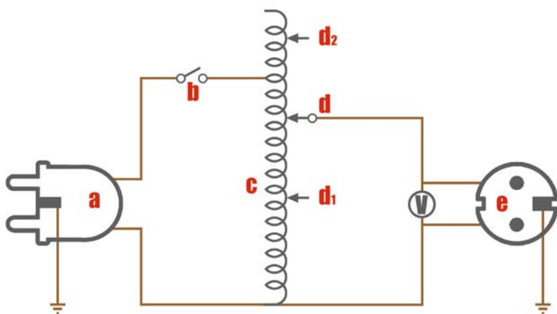
Bild 5: Variabler Transformator
