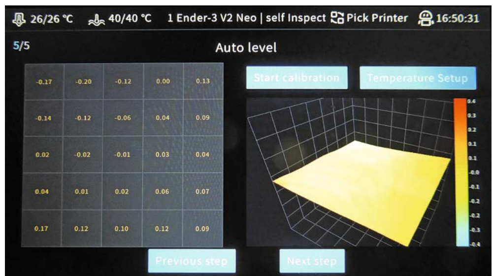
Bild 6: Mit der Autolevel-Funktion von KLIPPER lässt sich das Druckbett sehr exakt einstellen. Hier sieht man, dass an den Ecken noch nachgestellt werden muss.
