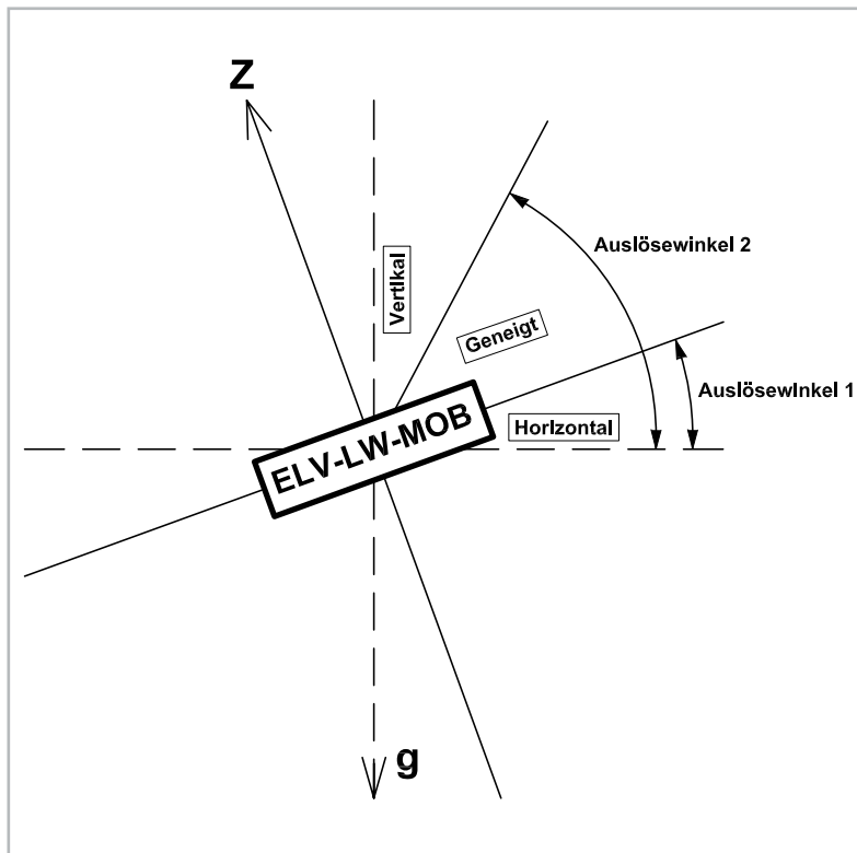
Bild 12: Die konfigurierbaren Auslöswinkel für die Lageerkennung (der Motion Button wird dabei von der Seite dargestellt, der App-Button befindet sich auf der Oberseite)
