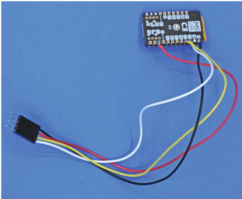
Bild 8: Verkabelung der ESP C3 Stamp
