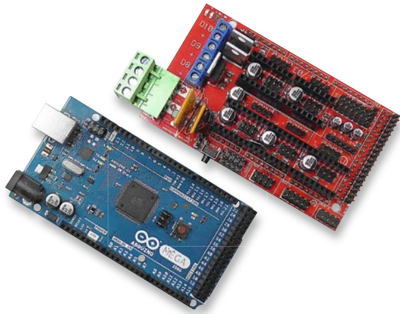
Bild 1: Ein typisches RAMPS-Shield für den Arduino Mega2560, hier fehlen nur noch die Schrittmotortreiber zur betriebsfertigen Steuerung für 3D-Drucker, CNC-Fräsen, Plotter etc.
