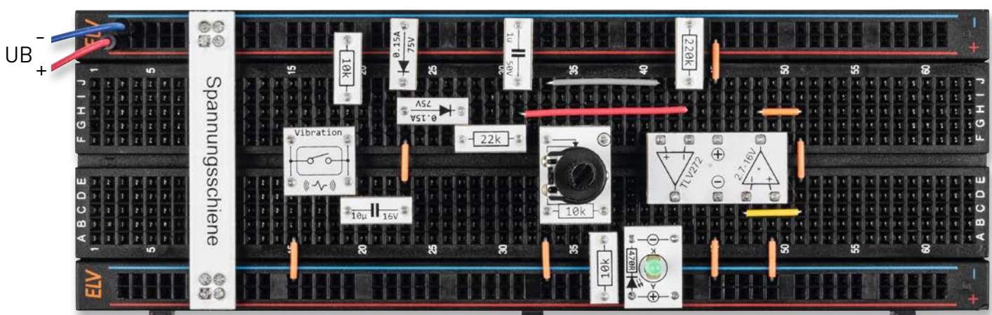
Bild 5: Beispielschaltung für einen Vibrationssensor, aufgebaut mit PAD-Komponenten
