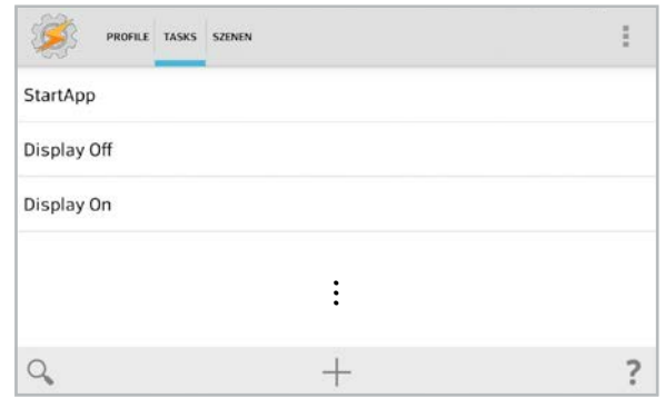
Bild 9: Task-Übersicht
