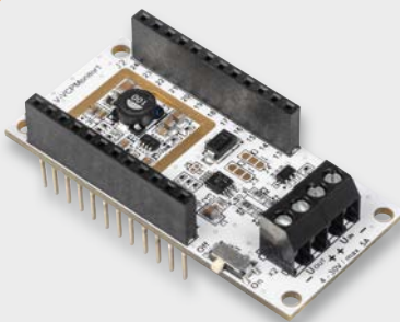
Applikationsmodul ELV-AM-VCPM1
