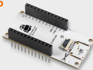
Applikationsmodul ELV-AM-LX1
