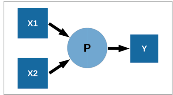
Bild 1: Perzeptron
