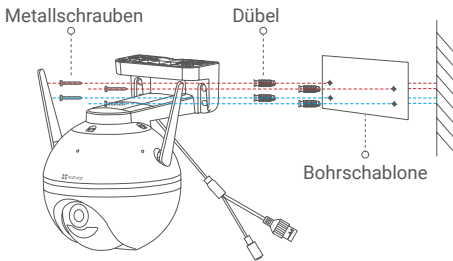
Abb. 1 Wandmontage
