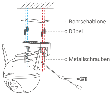
Abb. 2 Deckenmontage
