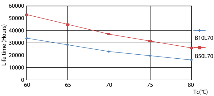
8W G13
