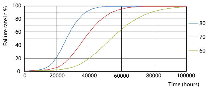
8W G13
