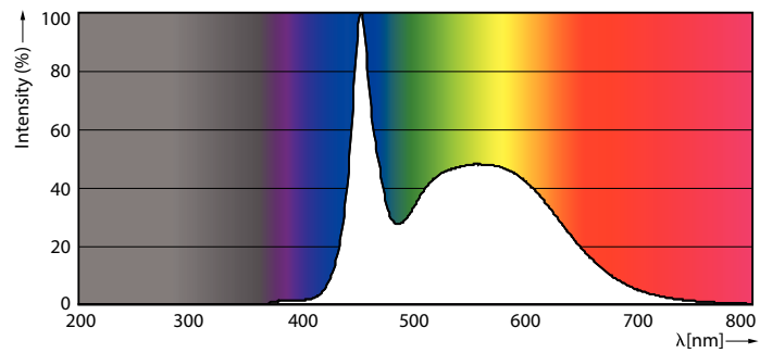
8W G13
