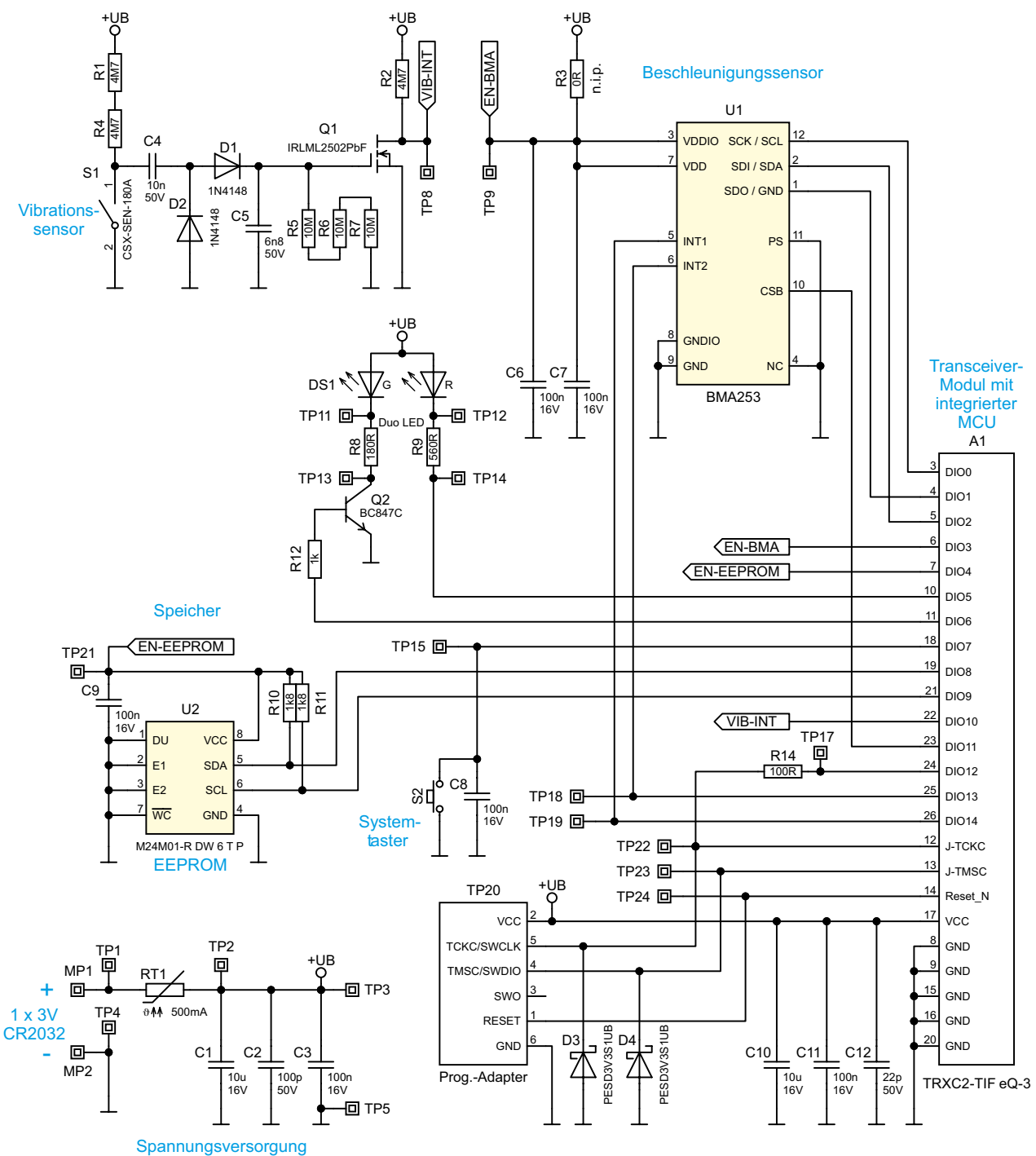
Bild 4: Das Schaltbild des HmIP-DLS
