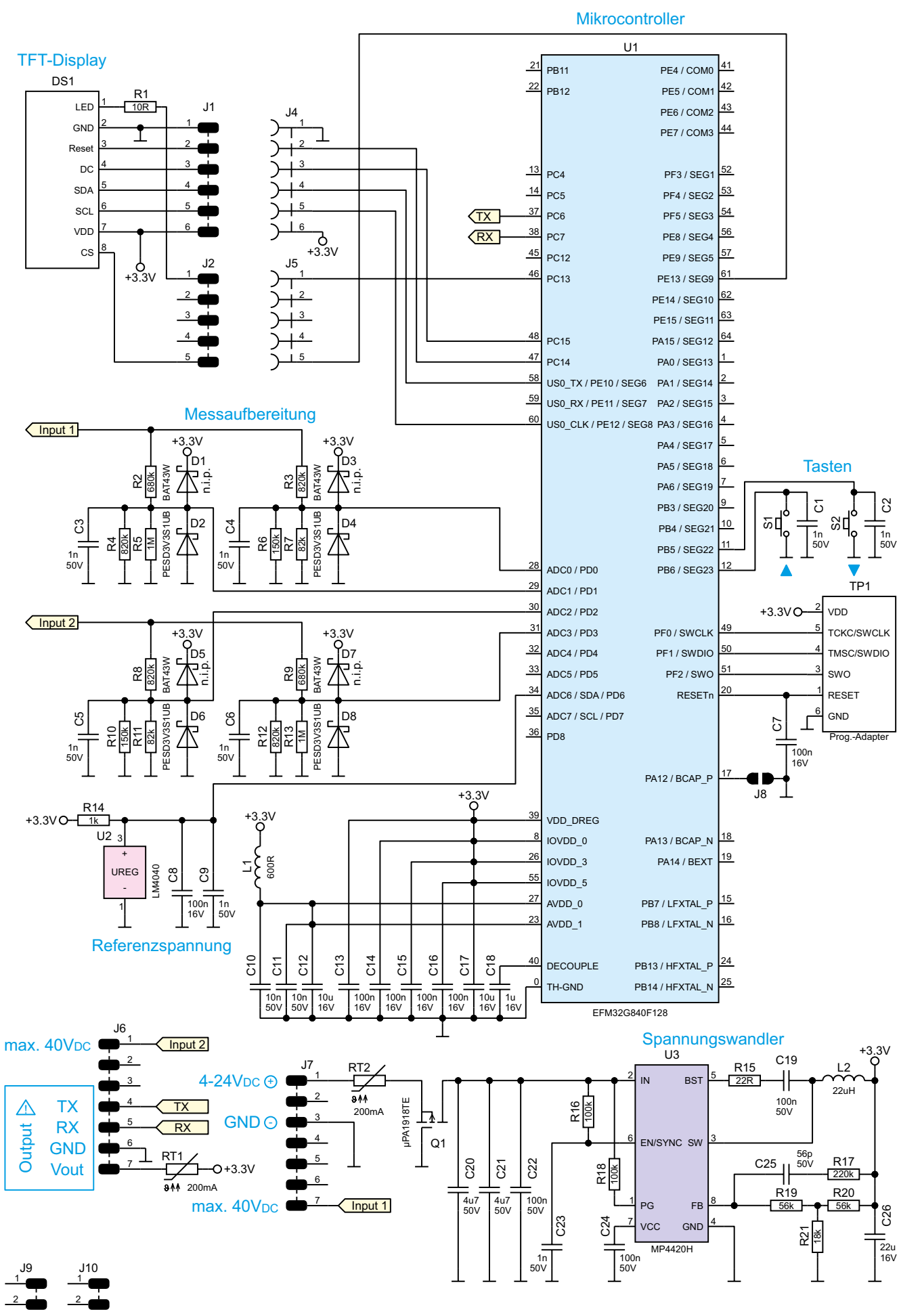
Bild 1: Schaltbild des Mini-Voltmeters mit Display
