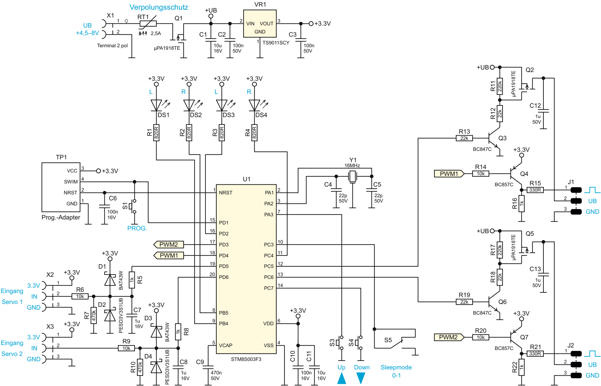
Bild 9: Schaltbild des Servo-Interface SIF1
