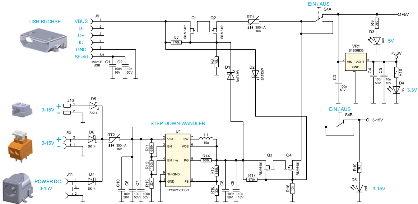
Bild 13: Schaltbild des EXSB-Mini
