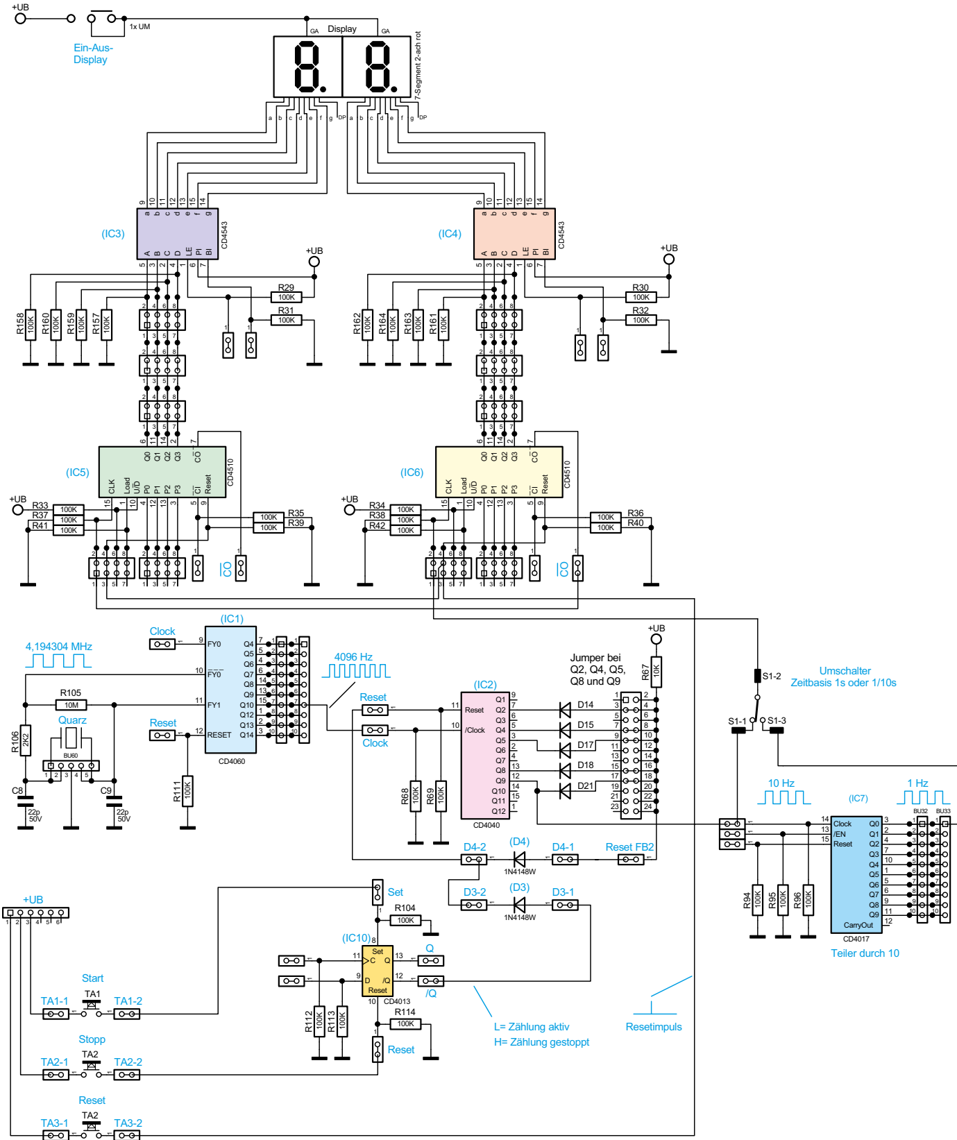
Bild 2: Verdrahtung auf dem DEB100 für die Stoppuhr
