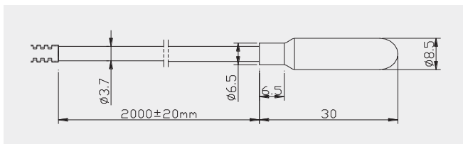
Technische Maßzeichnung Kunststoff-Tempersensoren TS2-2
