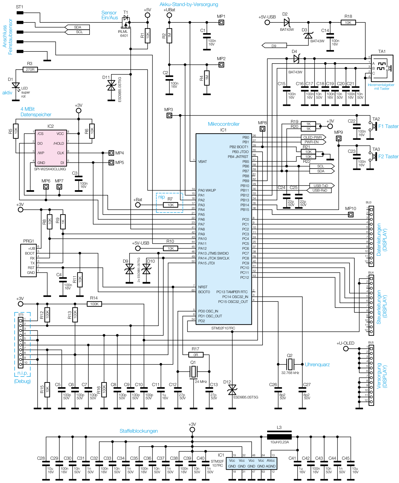
Bild 18: Mikrocontroller-Einheit des Feinstaub-Messgeräts PM2.5
