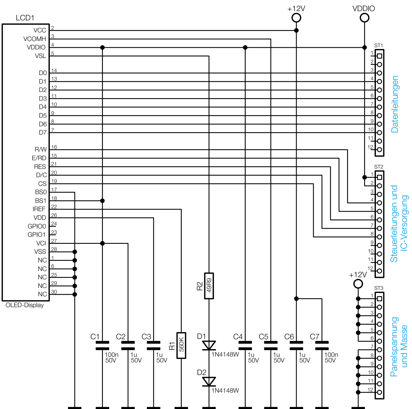
Bild 19: OLED-Displayeinheit
