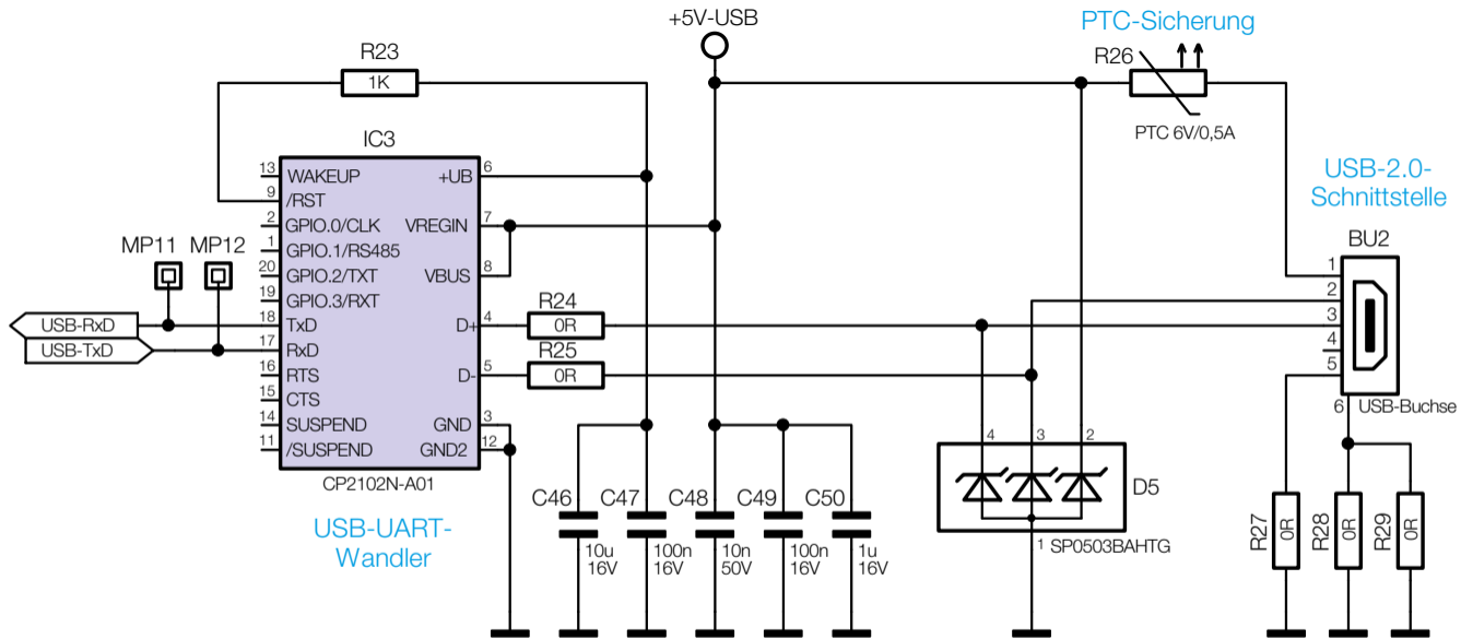
Bild 20: USB-Schnittstelle des Feinstaub-Messgeräts PM2.5
