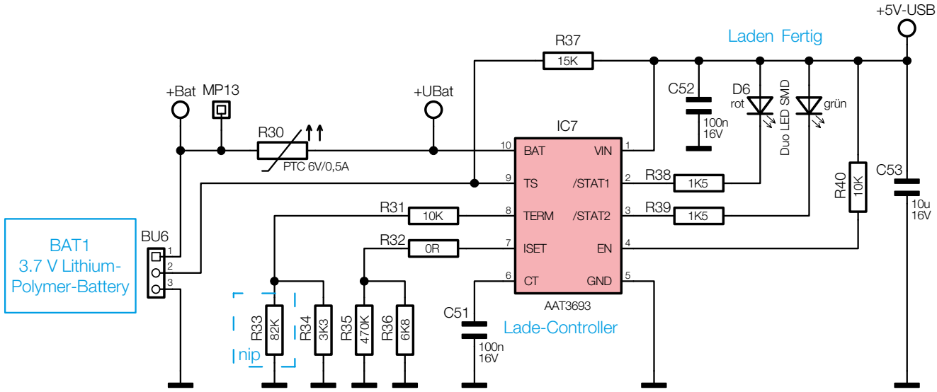
Bild 16: Lithium-Akku-Ladeschaltung
