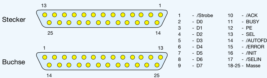
Parallel-Schnittstelle, DB 25 Stecker und Buchse, Sicht auf Lötanschlüsse
