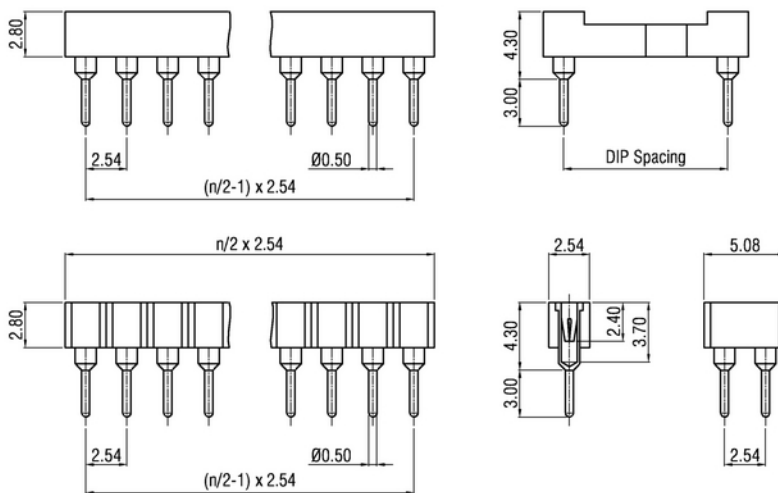
IC Socket Header 182
