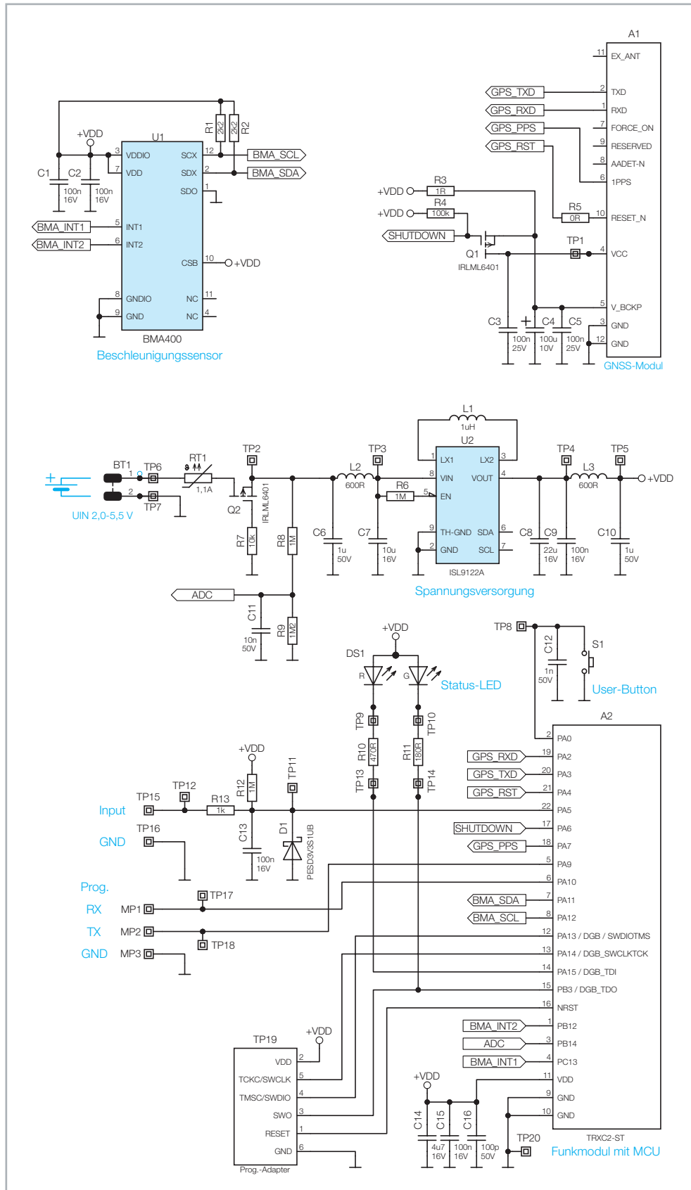
Bild 4: Das Schaltbild des ELV-LW-GPS2
