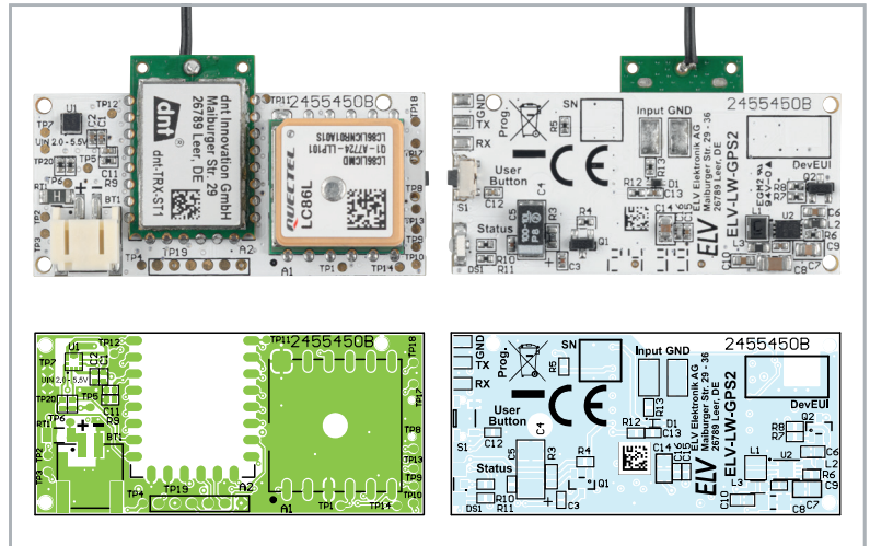
Bild 5: Platinenfotos und Bestückungsdrucke des ELV-LW-GPS2
