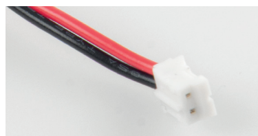
Bild 1: Stecker JST PH mit einem Rastermaß von 2 mm
