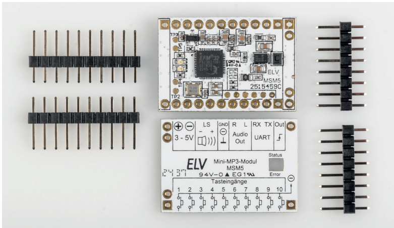
Bild 7: Lieferumfang
