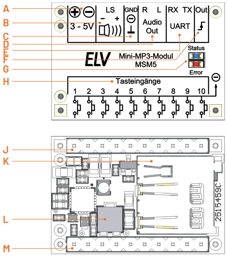
Bild 2: Geräteübersicht
