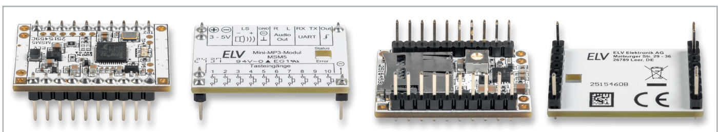
Bild 11: Eingelötete Stiftleisten
