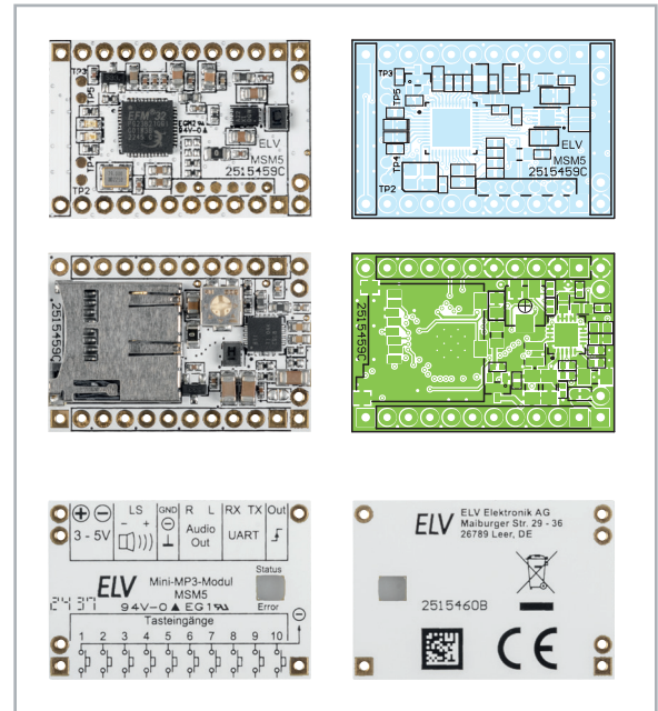
Bild 8: Vorder- und Rückseite der beiden Platinen (Originalgröße)
