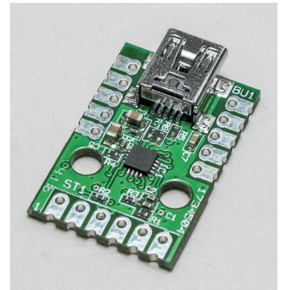
Bild 4: USB-UART-Wandler UM2102N
