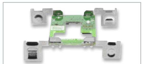
Bild 5: Die Batteriekontakte müssen genau senkrecht zur Platine stehen.
