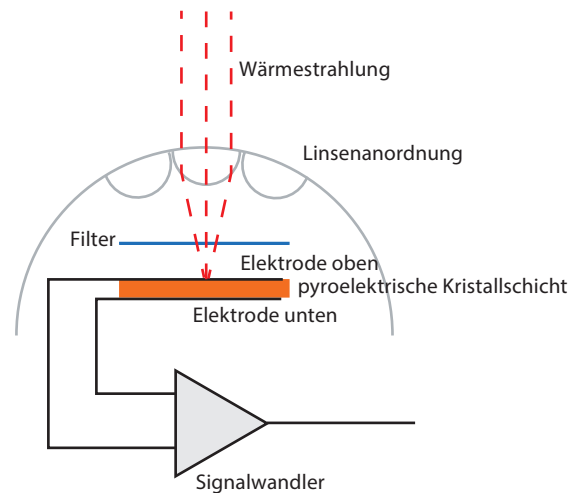
PrinzipaufbaueinesBewegungsmelders
