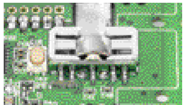
Bild 12: So wird die Sensorplatine mit der Basisplatine verlötet. Dabei sind Lötzinnbrücken zwischen den einzelnen Kontakten zu vermeiden.
