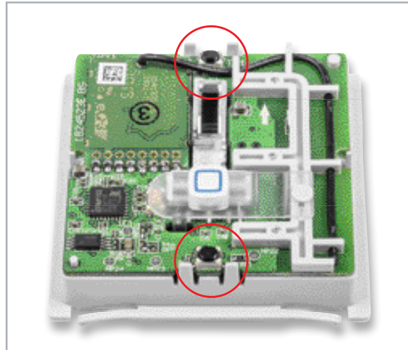
Bild 17: Nach dem Einsetzen der Basisplatine in die Batterieplatte muss die Basisplatine an den gekennzeichneten Rastnasen einrasten.
