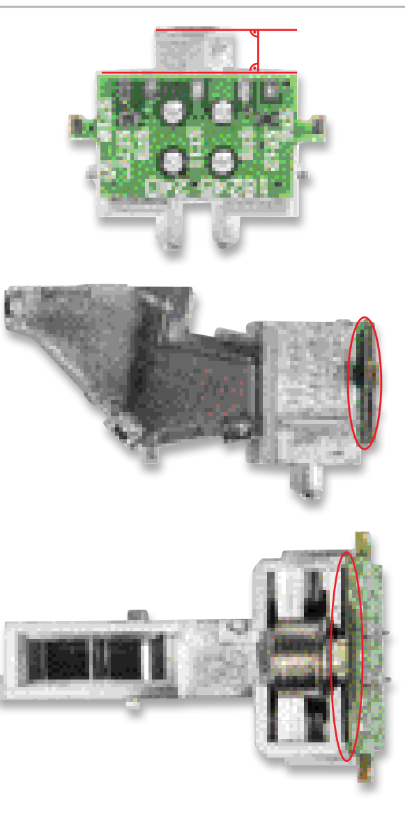
Bild 7: Die Sensoroptik muss exakt plan auf der Sensorplatine aufliegen.
