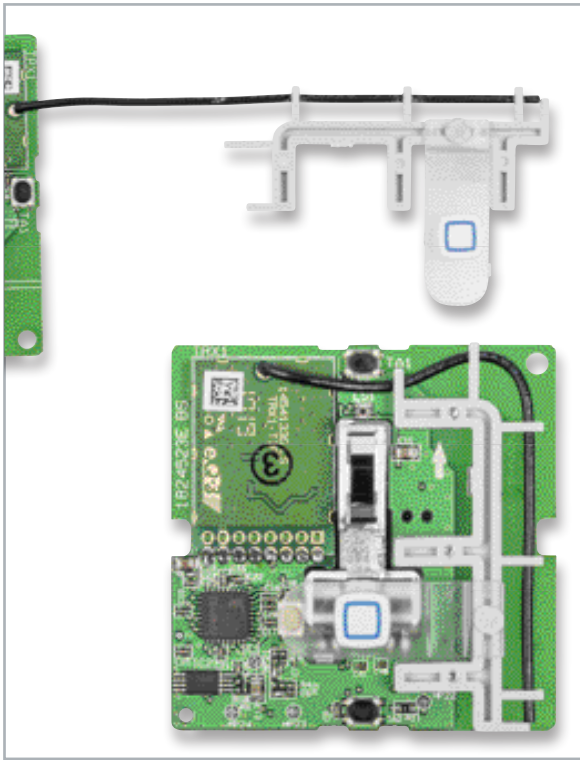
Bild 13: Die Antenne wird, mit ihrem Ende beginnend, in den Antennenträger eingesteckt und der Antennenträger mittels dreier Schrauben auf der Basisplatine befestigt.
