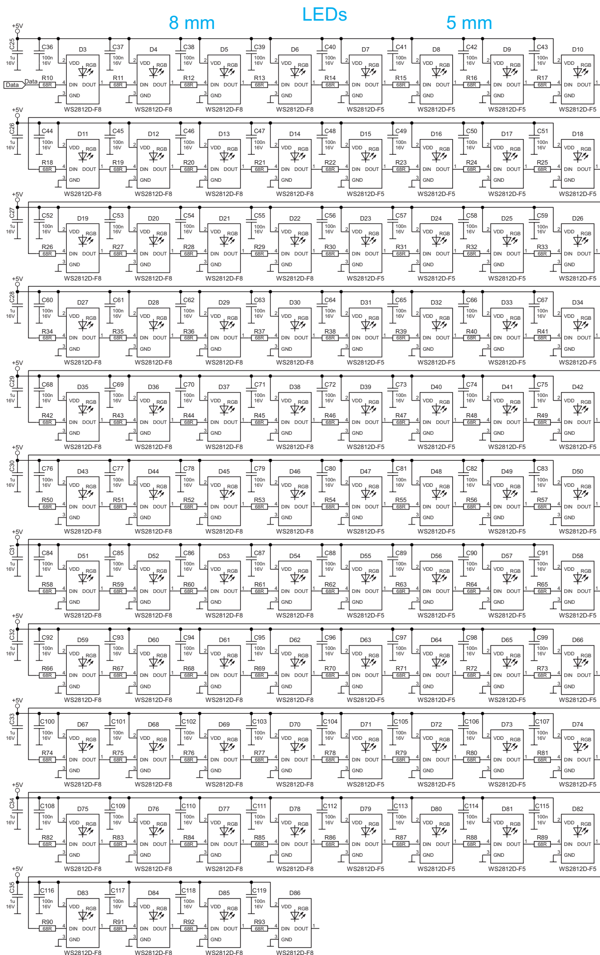
Bild 3: Schaltbild WS2812-LEDs
