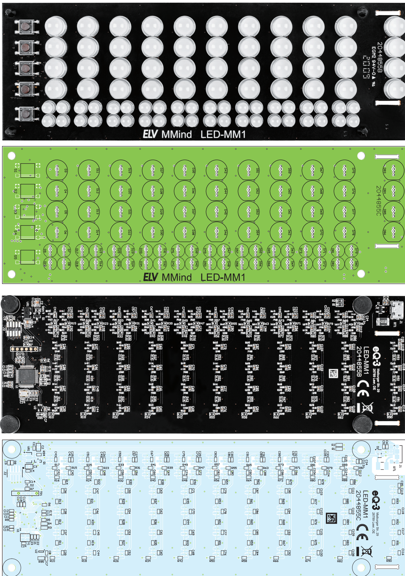
Bild 4: Platinenfotos und Bestückungspläne von der Bestückungsseite (oben) und der Lötseite (unten)
