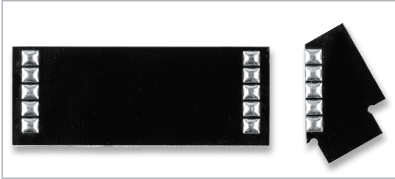
Bild 9: Die Pads vor der Montage verzinne
