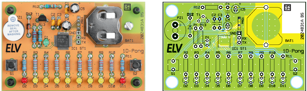
Bild 3: Platinenfoto des komplett bestückten 1D-Pong mit dem zugehörigen Bestückungsplan
