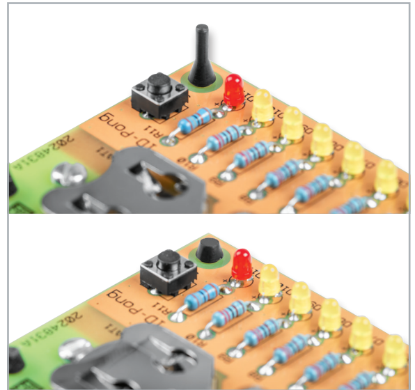
Bild 12: Hier ist ein durchgesteckter (oben) und gekürzter (unten) Gummifuß zu sehen.
