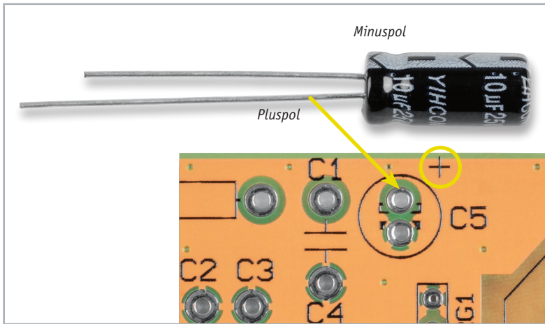
Bild 11: Die Polaritätsmarkierungen des Elektrolyt-Kondensators und die zugehörige Platzierungsmarkierung auf der Platine
