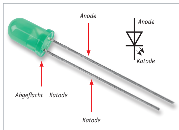
Bild 8: So identifiziert man Anode und Katode der Leuchtdioden.
