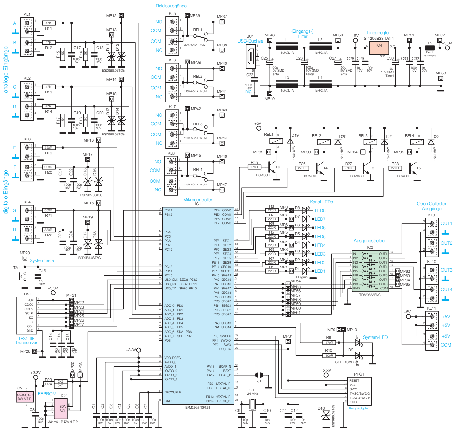
Bild 1: Schaltbild der Homematic IP Multi-IO-Modulplatine – 4 x 4
