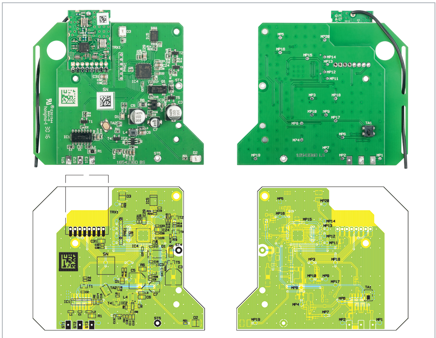
Bild 2: Platinenfoto und Bestückungsplan der fertig bestückten Platine
