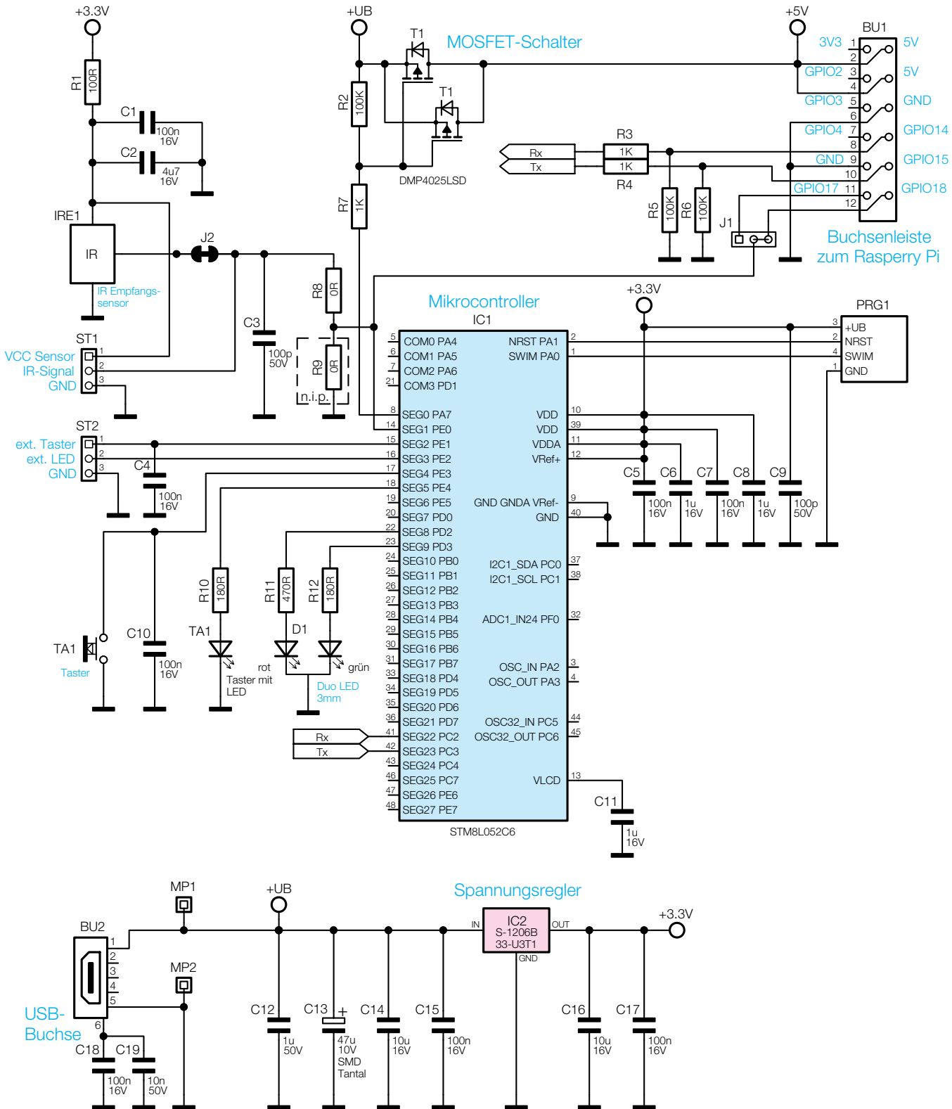
Bild 1: Das Schaltbild des Raspberry-Pi-Power-Controllers RPi-PC
