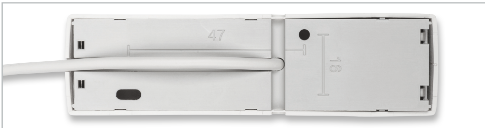
Bild 9: Das Verbindungskabel zum Kontakt wird, wie hier gezeigt, durch einen der Kabelkanäle auf der Geräterückseite und die zugehörige Bohrung in das Gehäuse geführt. Hier ist auch das entsprechend vorbereitete Gehäuseoberteil aufgesetzt.
