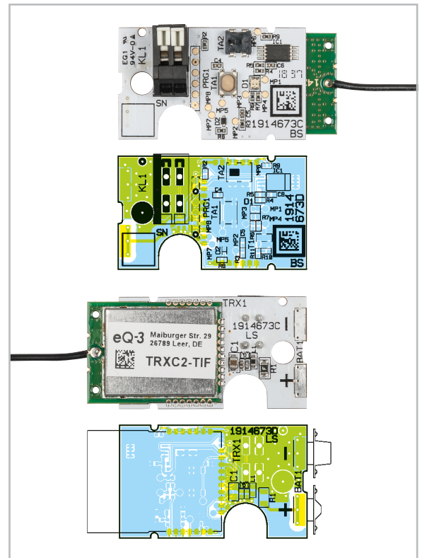
Bild 3: Die Platinenfotos des HmIP-SCI mit den jeweils zugehörigen Bestückungsdrucken, oben die Oberseite mit Taster und Anschlussklemme, unten die Unterseite mit TRX-MCU-Modul
