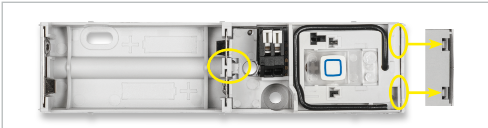
Bild 8: Der Antennenhalter ist im Bereich des Batteriehalters (Markierung links) einzusetzen und am hinteren Ende (hier rechten) Ende einzurasten (siehe Detailbild rechts). Hier ist auch die Lage der Antennen zu sehen.
