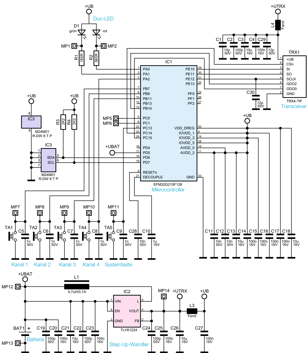
Bild 1: Das Schaltbild der Homematic IP Schlüsselbundfernbedienung
