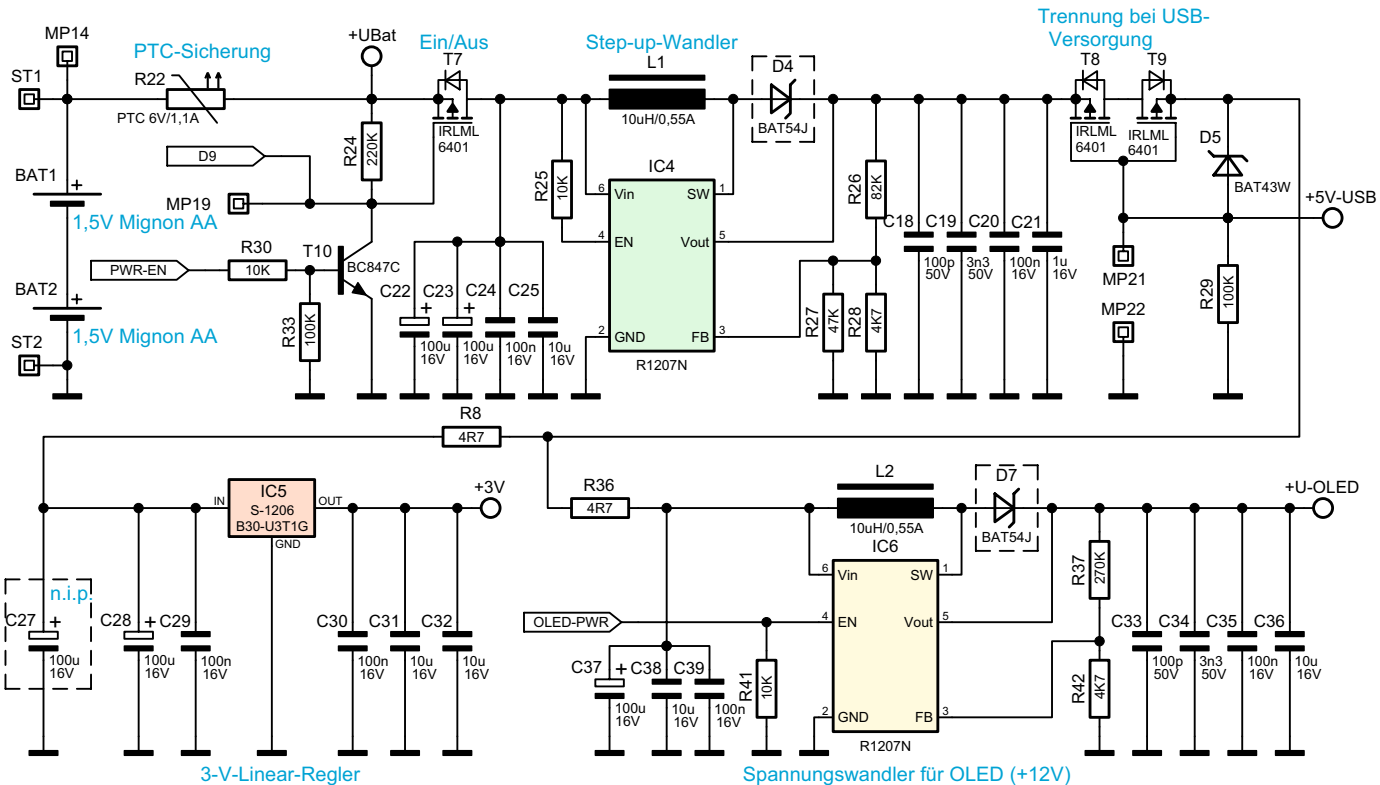
Bild 15: Spannungsversorgung des RGBW200
