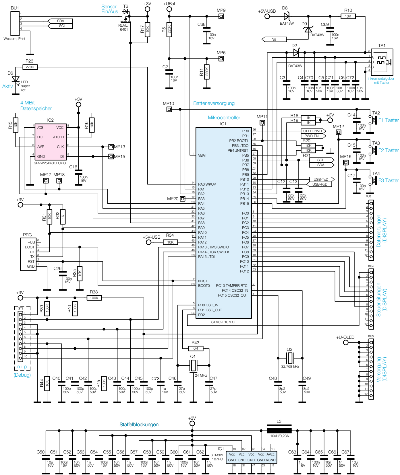
Bild 16: Mikrocontroller-Einheit des RGBW200
