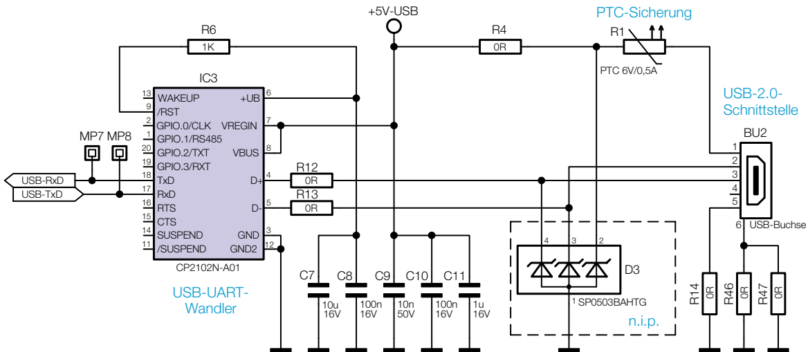
Bild 19: USB-Schnittstelle des RGBW200
