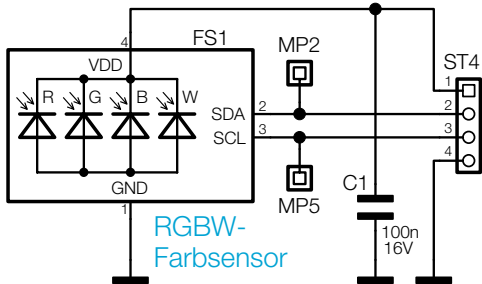
Bild 18: Sensoreinheit des RGBW200
