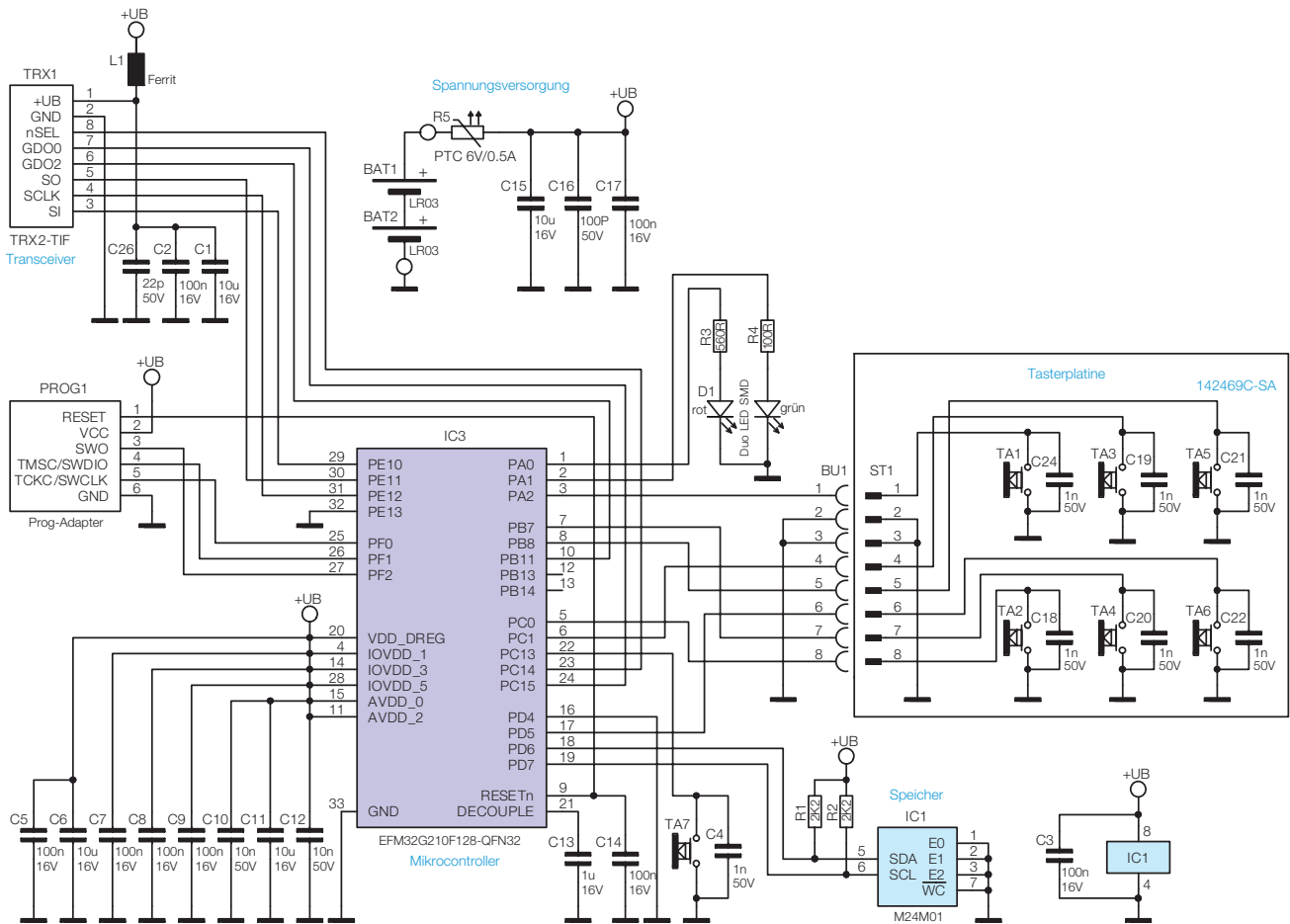
Bild 1: Das Schaltbild des Homematic IP 6fach Funk-Wandtasters
