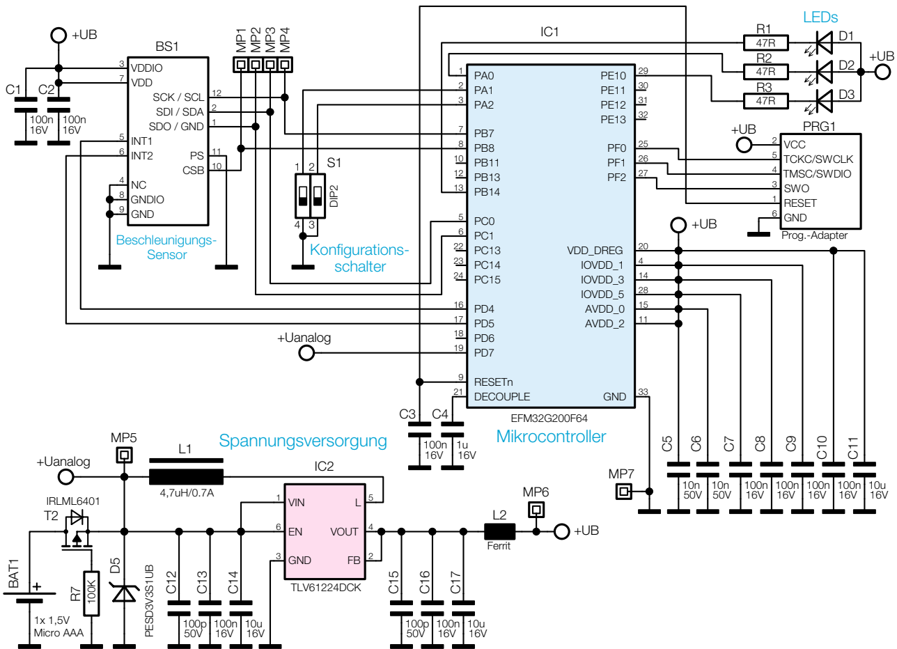
Bild 1: Das Schaltbild des ES100
