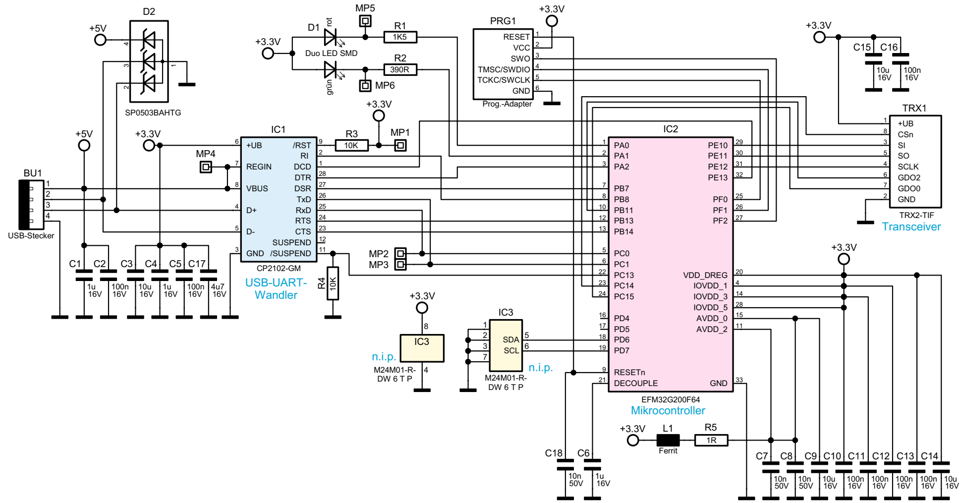
Bild 1: Das Schaltbild des HmiTP-RFUSB
