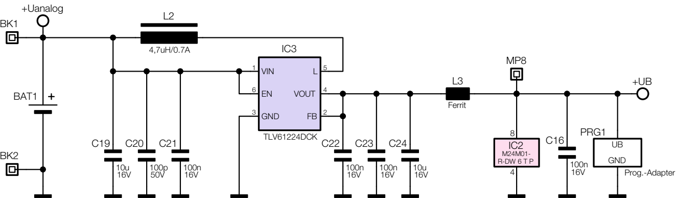
Bild 2: Das Schaltbild des Fenstergriffsensors HmIP-SRH
