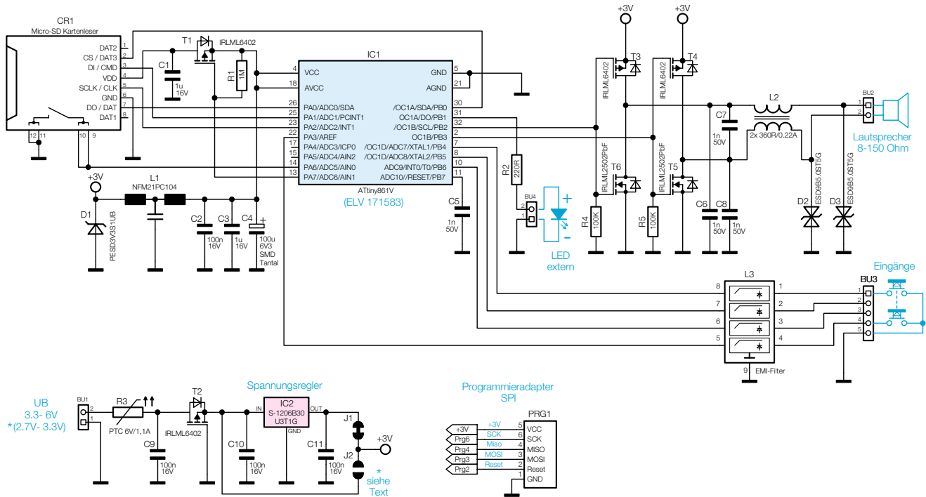
Bild 2: Schaltbild des Mini-Wave-Players
