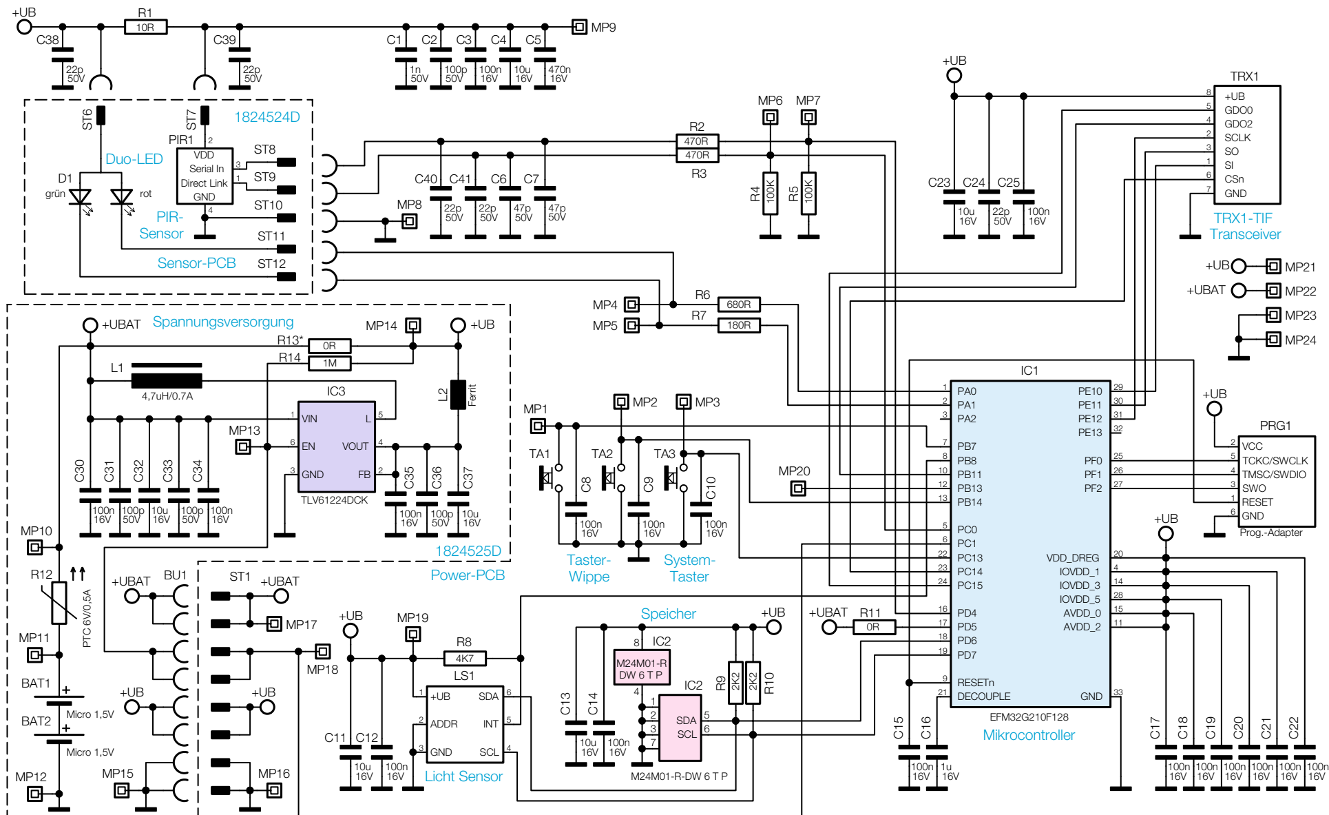
Bild 1: Das Schaltbild des HmTP-SM155
