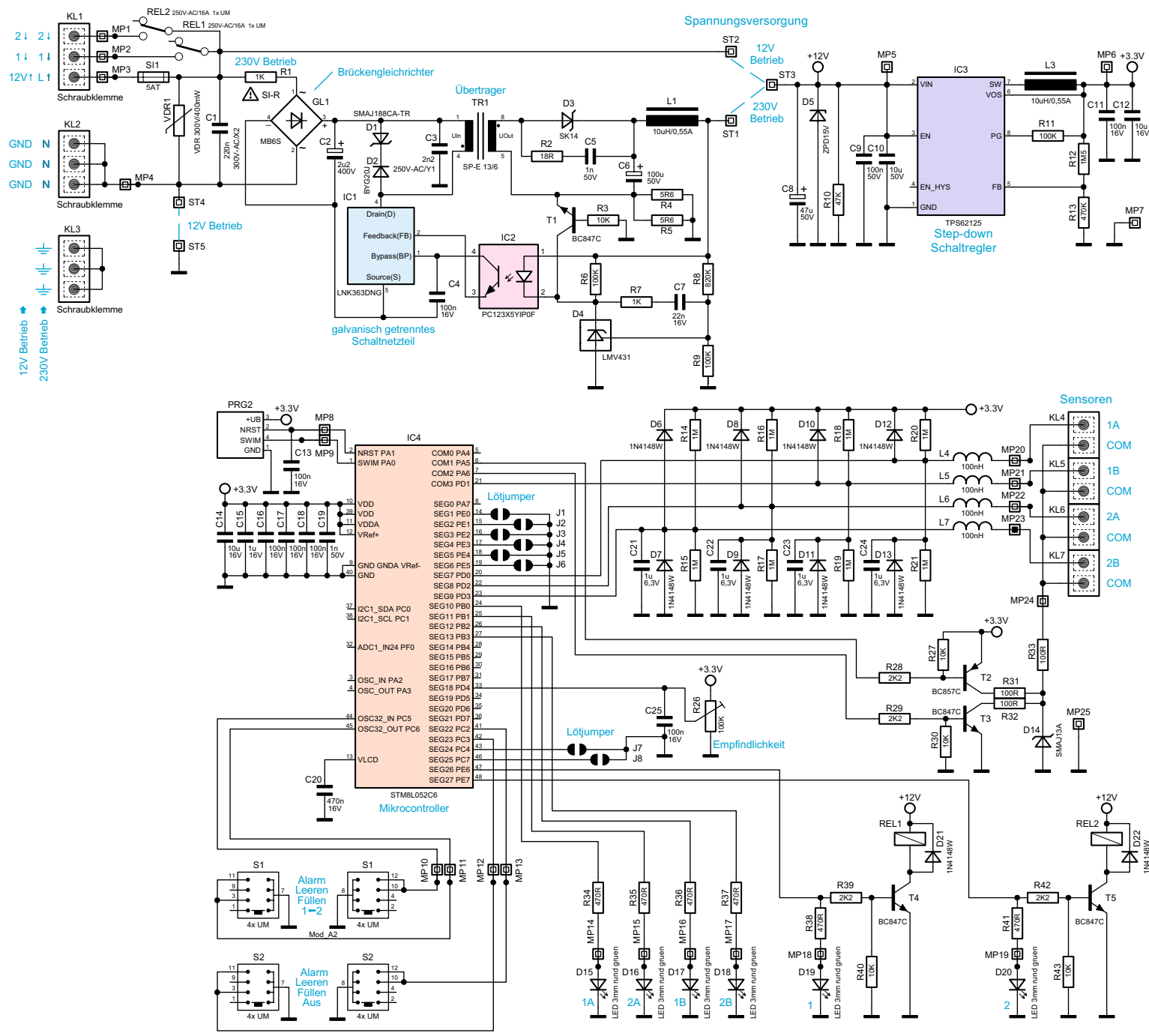
Bild 4: Das Schaltbild
