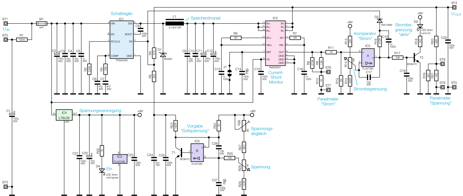
Bild 2: Gesamtschaltbild des SPM1505
