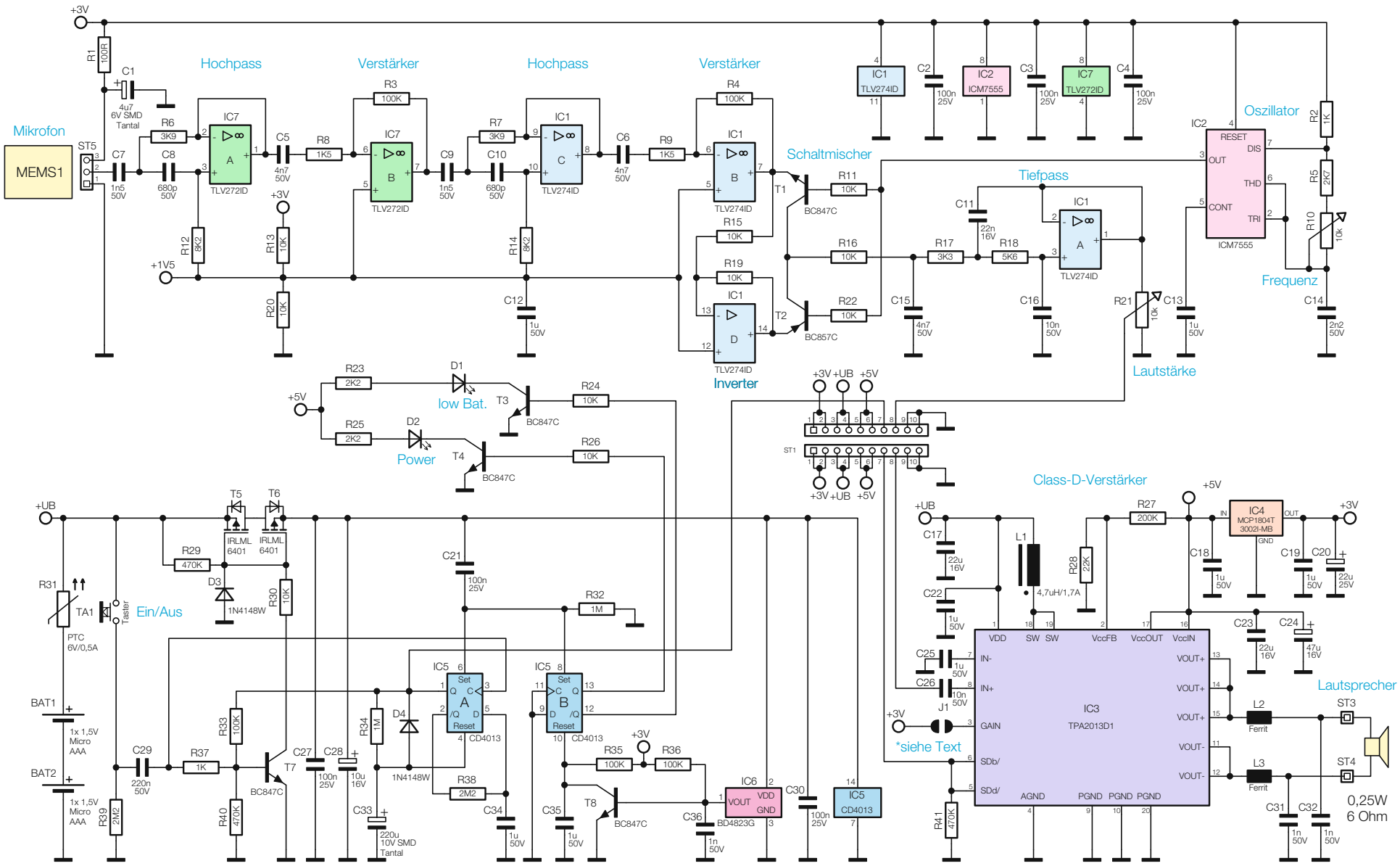
Bild 5: Das komplette Schaltbild des FMD1
