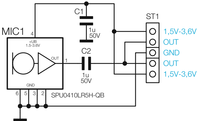
Bild 10: Das Schaltbild der MEMS-1-Platine
