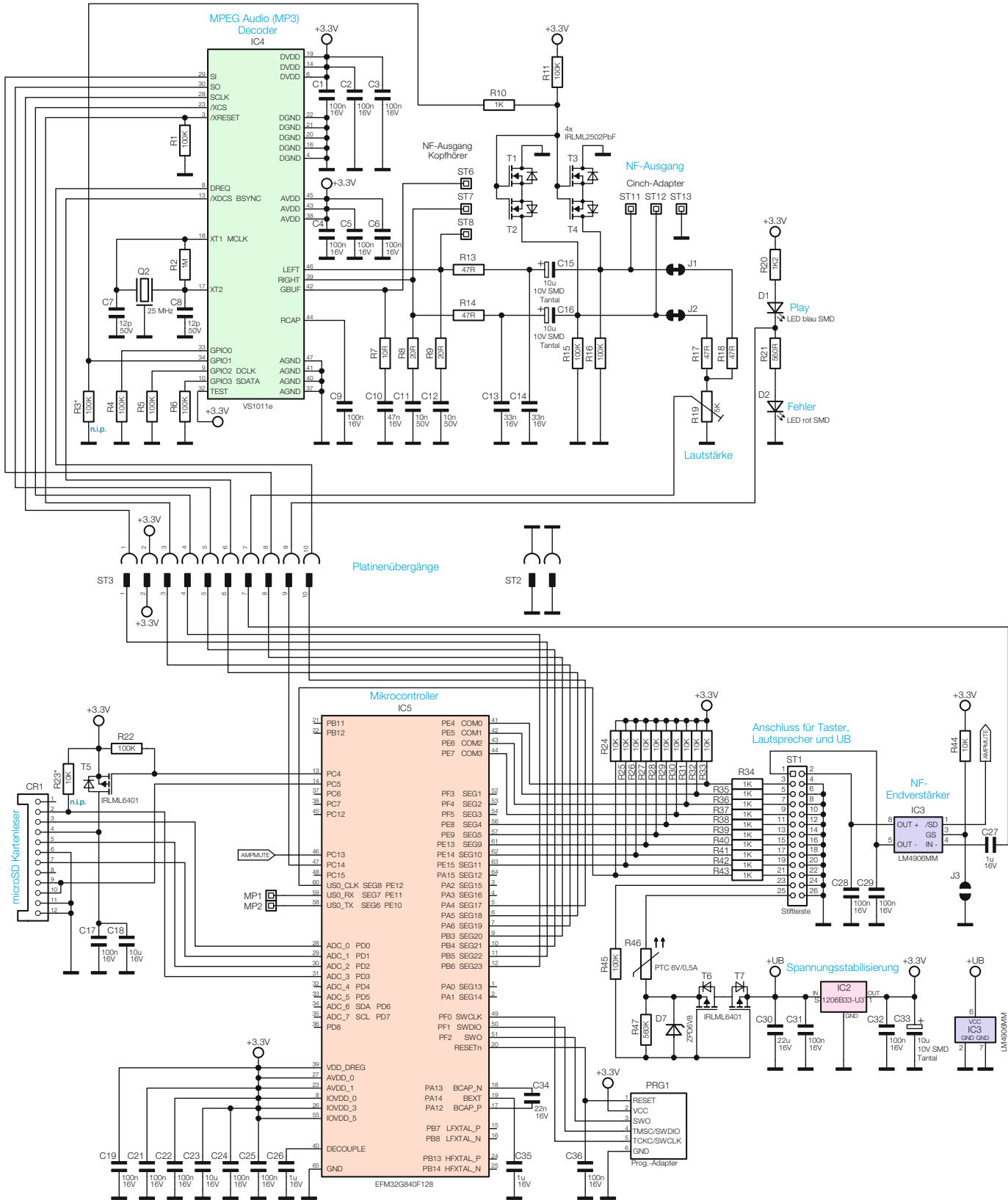
Bild 4: Das Schaltbild des MSM4
