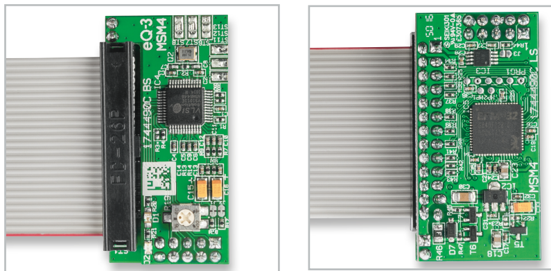
Bild 11: Sämtliche Anschlüsse des MP3-Soundmoduls können über einen Flachbandkabel-Steckverbinder hergestellt werden.
