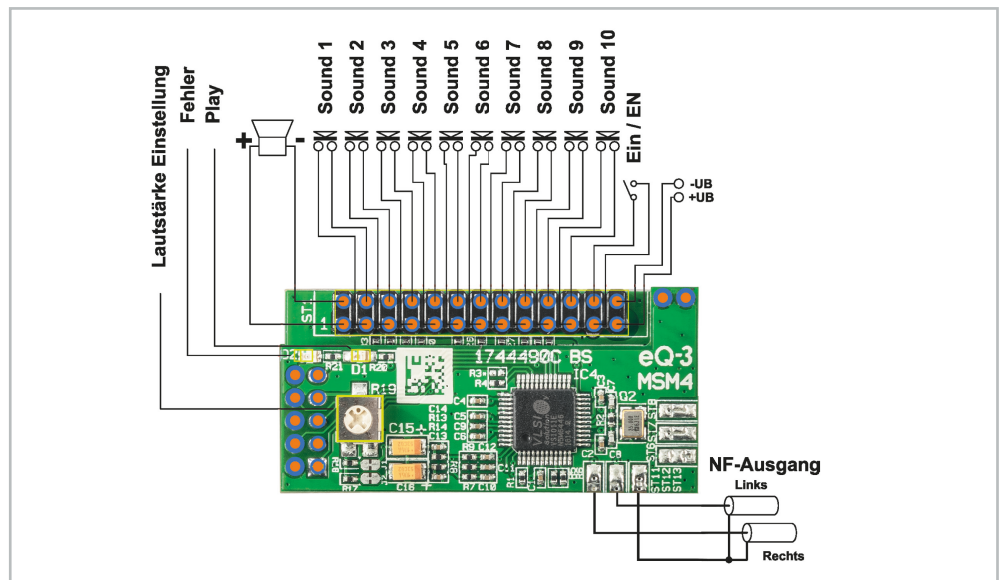
Bild 1: Bedien- und Anzeigeelemente sowie die Anschlussbelegung des MP3-Soundmoduls
