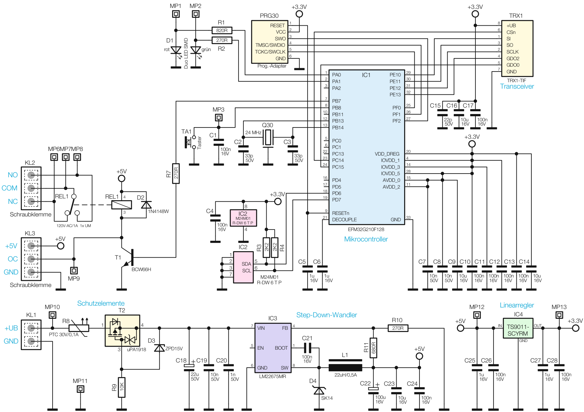
Bild 1: Das Schaltbild des Schaltaktors HmiTP-PCBS
