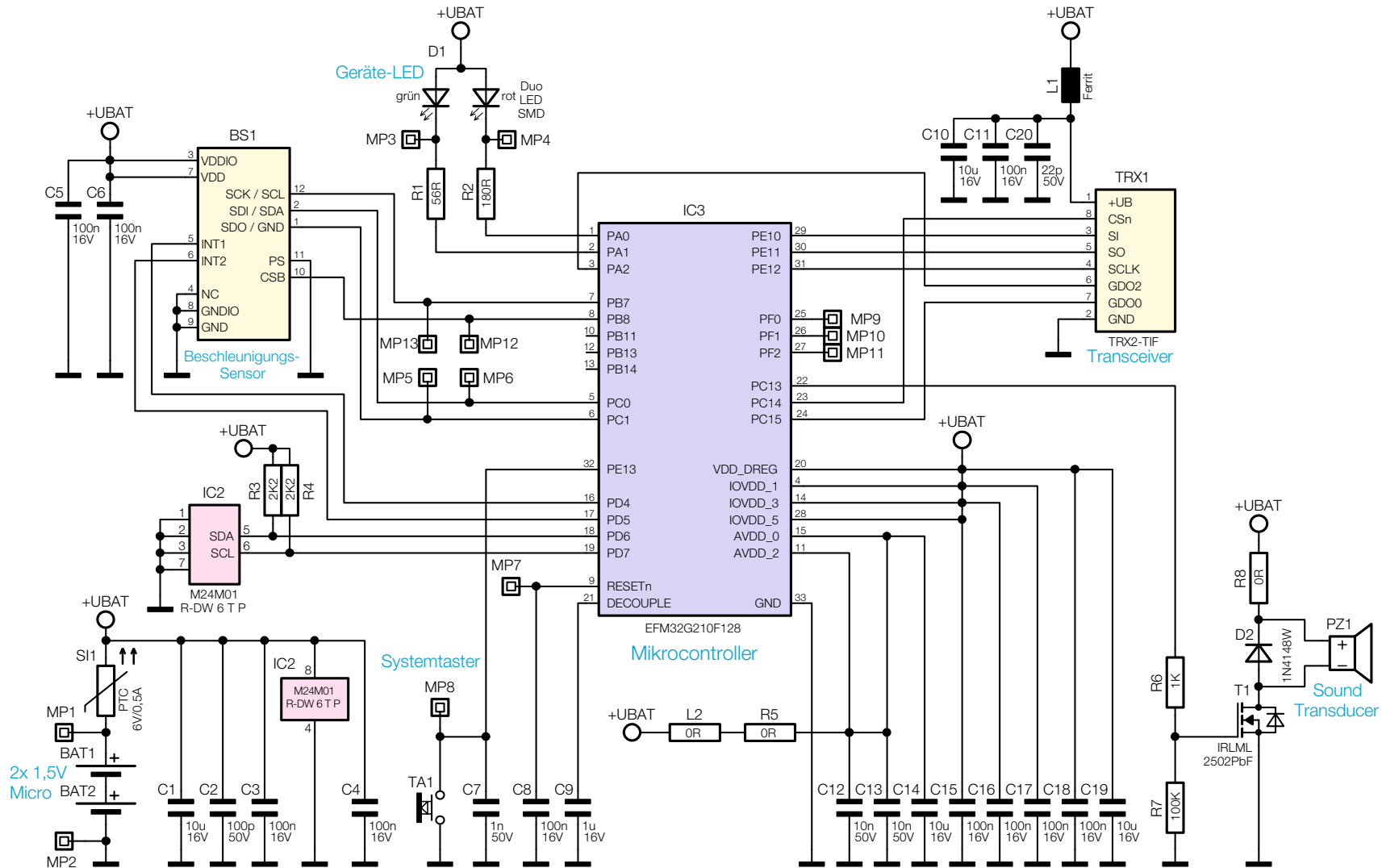
Bild 4: Das Schaltbild des HmTP-SAW
