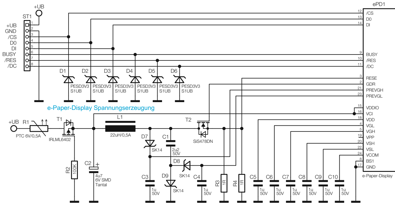
Bild 1: Das Schaltbild des E-Paper-Display-Moduls
