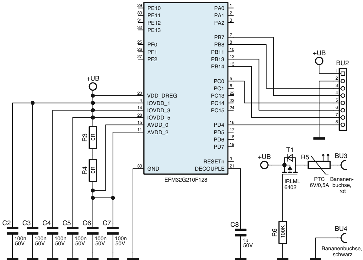
Bild 11: Das EFM32-Demoboard-Schaltbild
