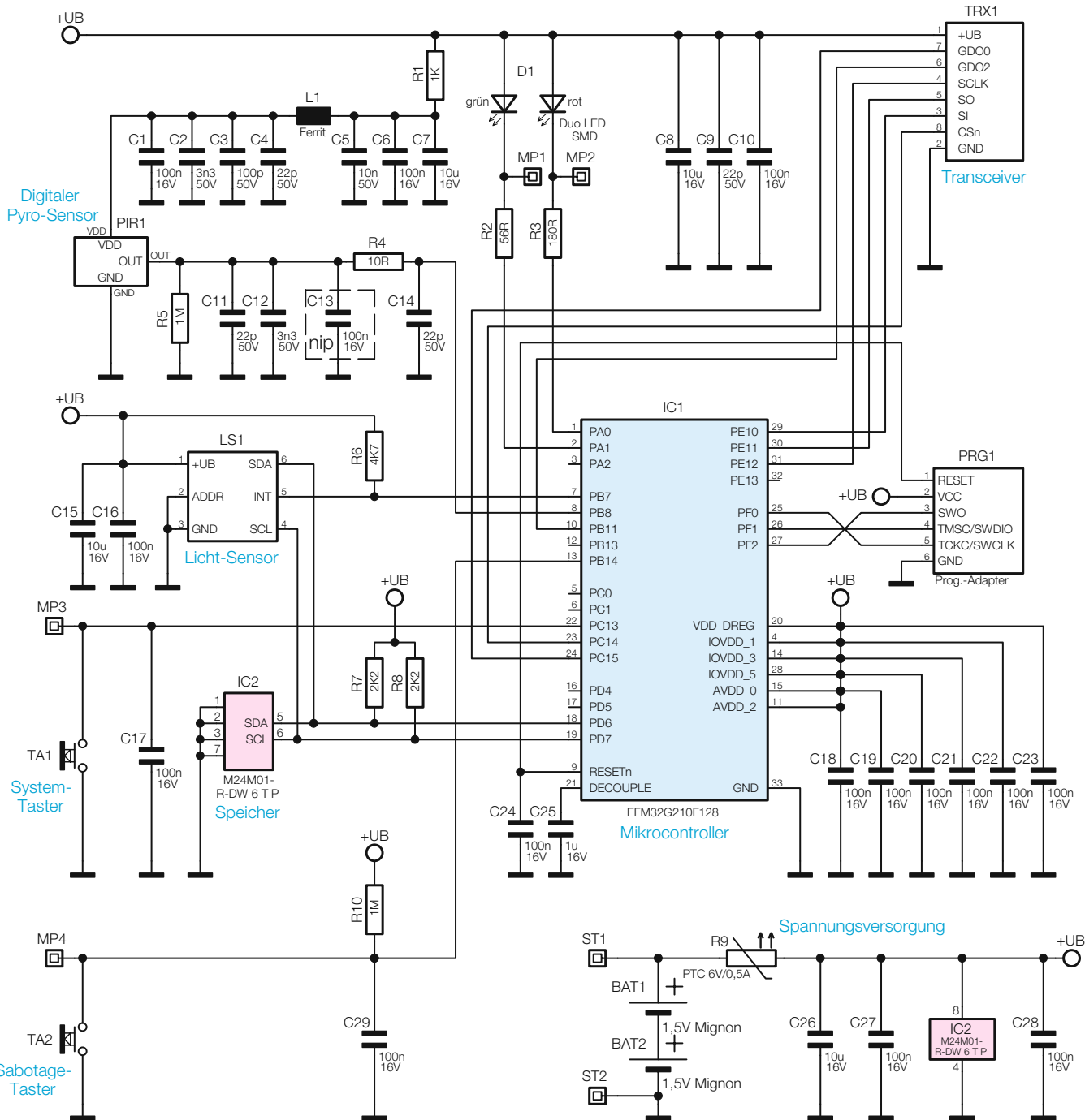
Bild 3: Das Schaltbild des Bewegungsmelders mit Dämmerungssensor
