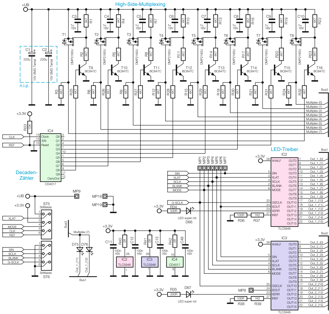
Bild 3: Schaltbild des High-Side-Multiplexing und der LED-Treiber
