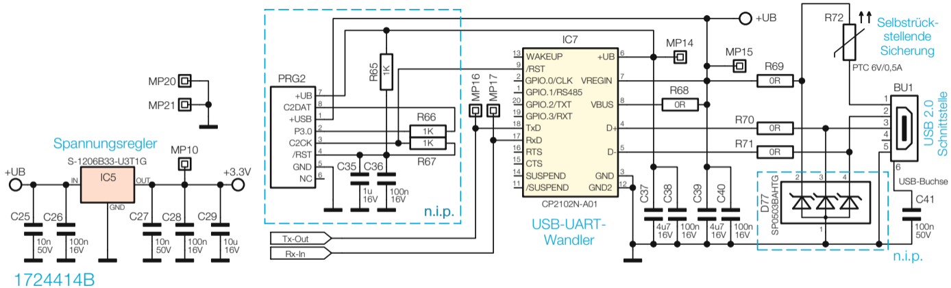
Bild 1: Schaltbild der Spannungsversorgung und des USB-Wandlers des KWL1
