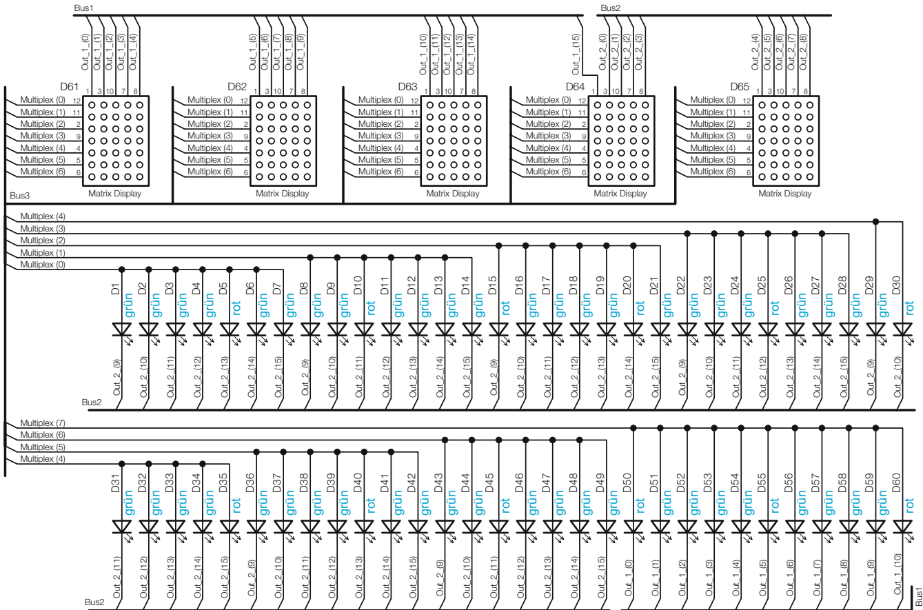
Bild 4: Schaltbild der einzelnen LED-Anschlüsse
