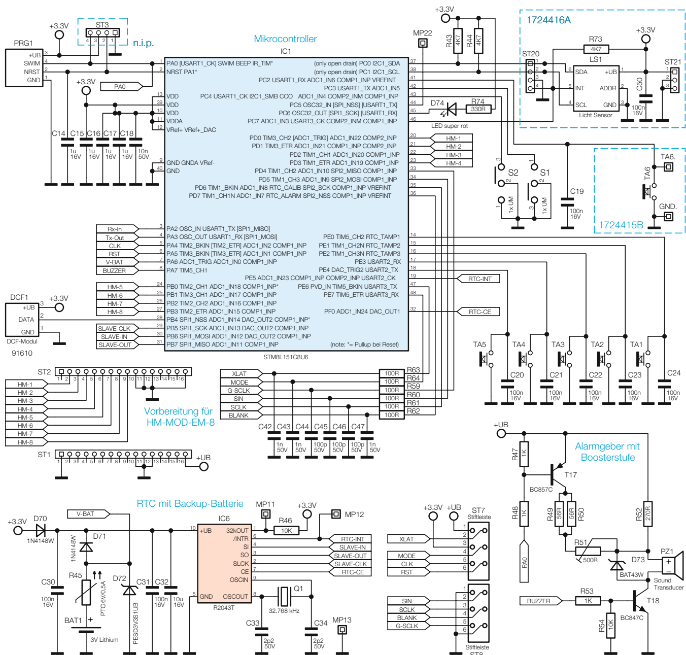
Bild 2: Schaltbild des Mikrocontrollers und der angeschlossenen Peripherie
