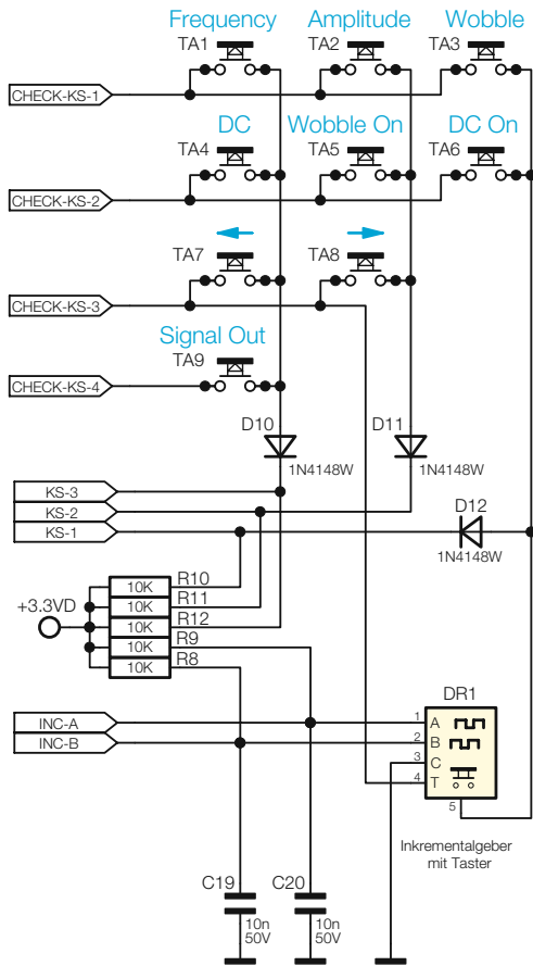
Tastenmatrix und Inkrementalgeber
