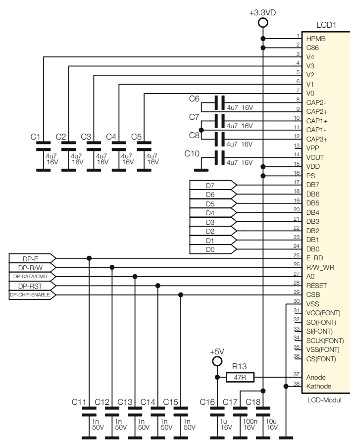
Display-Steuerleitungen
