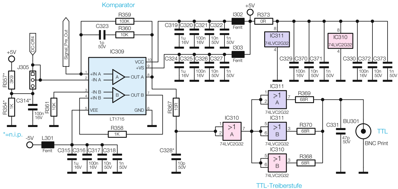
Bild 8: Der Komparator mit der TTL-Treiberstufe
