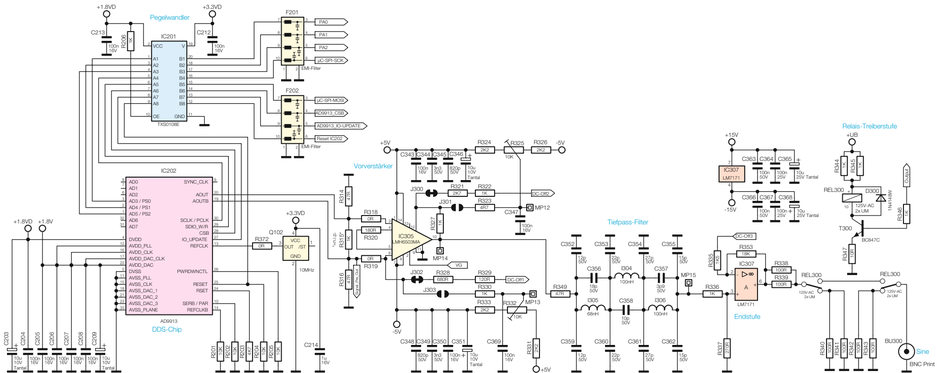
Bild 7: Schaltbild der DDS-Signalerzeugung mit dem Vorverstärker, dem Filter und der Endstufe
