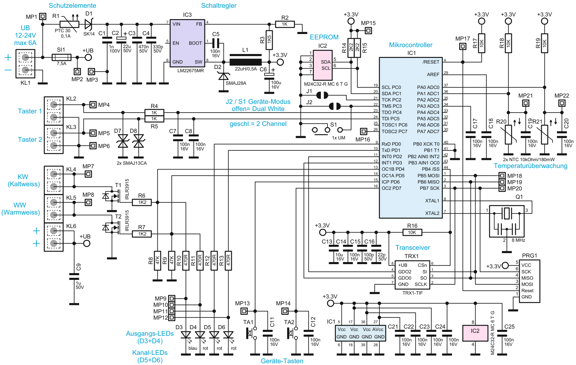
Bild 11: Das Schaltbild des Dual-White-Controllers
