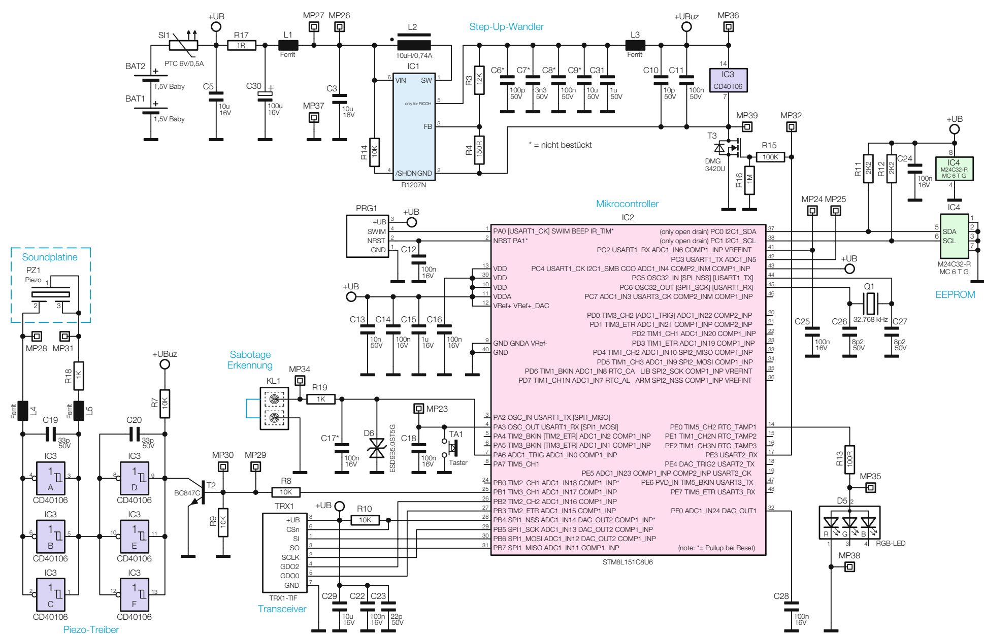
Bild 3 : Das Schaltbild der Sirene
