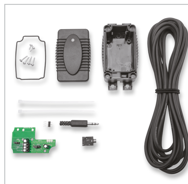
Bild 6: Der komplette Lieferumfang des Bausatzes zum hinzuzufügenden Empfangsmodul
