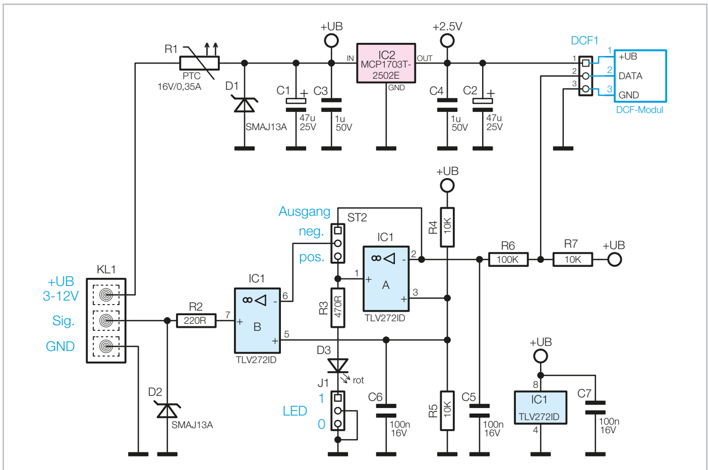
Bild 3: Das Schaltbild der DCF-ET1: Oben ist die Spannungsversorgung zu sehen, darunter die Signalaufbereitung.
