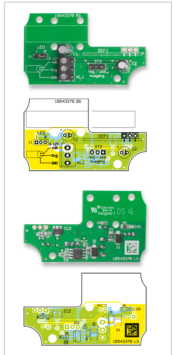
Bild 5: Die Platinfotos und die Bestückungspläne des DCF-Moduls: oben die Oberseite mit bedrahteten Bauteilen, unten die Unterseite mit SMD-Bestückung
