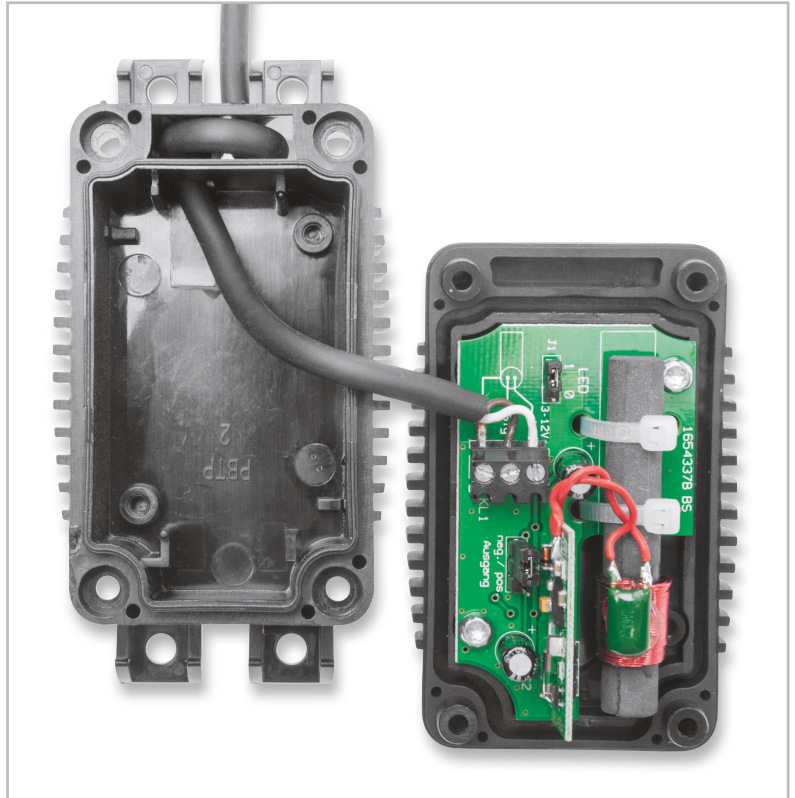
Bild 10: Die fertig montierte und mit Kabel versehene Einheit kurz vor dem Zusammenbau des Gehäuses
