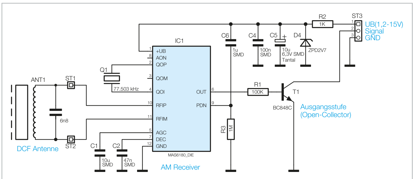
Bild 4: Das Schaltbild des ELV-Empfangsmoduls DCF-2 (Art.-Nr. 09 16 10)
