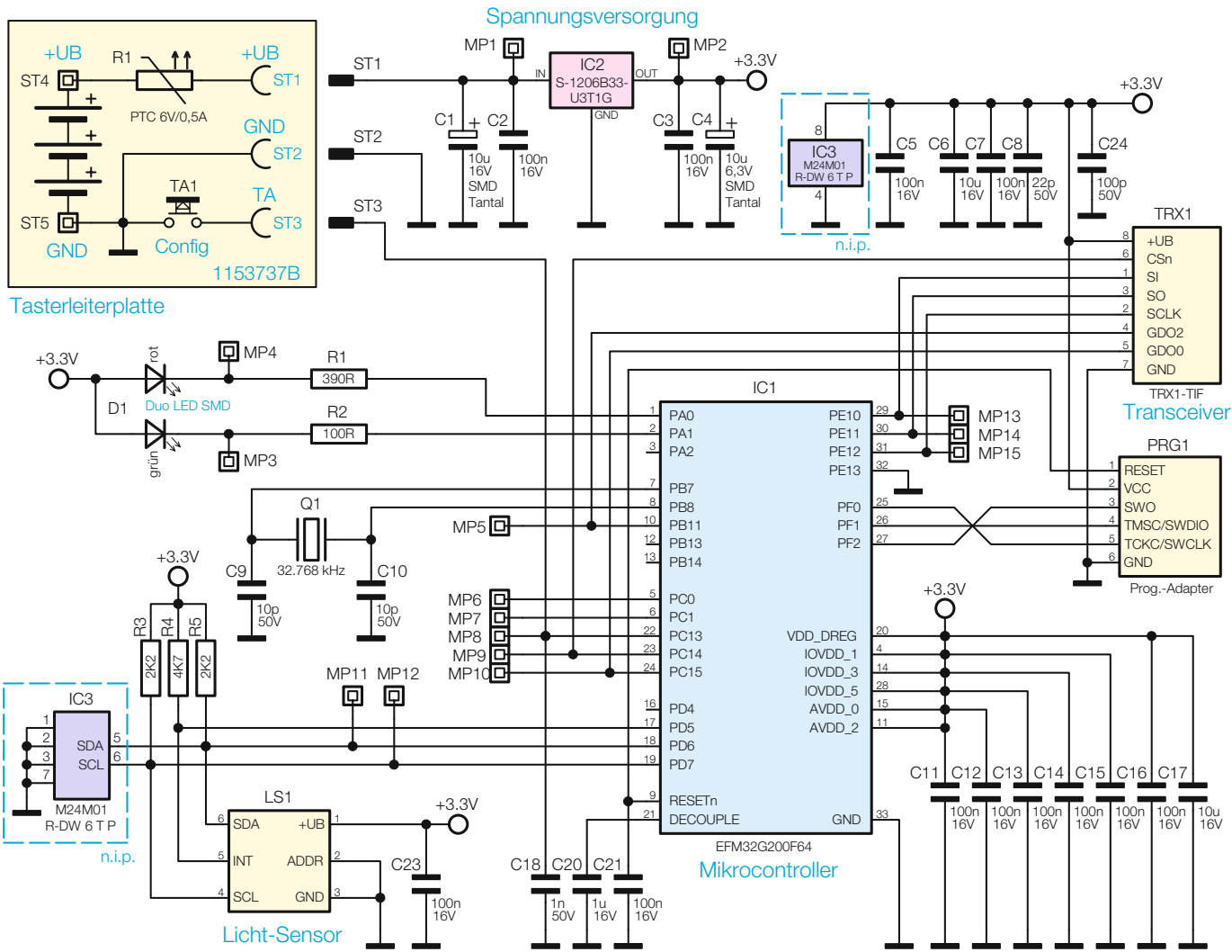
Bild 1: Das Schaltbild des Lichtsensors HM-Sen-LI-0
